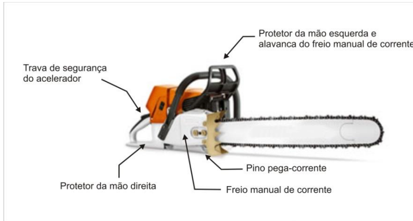
Figura 6: dispositivos de segurança obrigatórios de uma motosserra.
