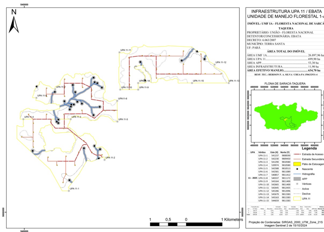
Figura 5: Infraestrutura a ser implantada na UPA 11/2025, UMF 1A, Floresta Nacional Saracá-Taquera (Lote-Sul), Terra Santa, Pará.
