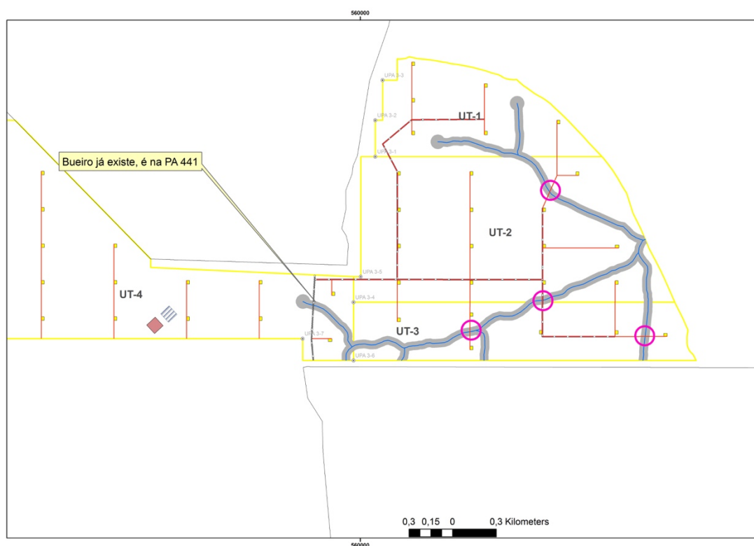
Figura 6: Infraestrutura de bueiros a ser implantada na UPA 3/2017, UMF 1A, Floresta Nacional Saracá-Taquera (Lote-Sul), Terra Santa, Pará.
