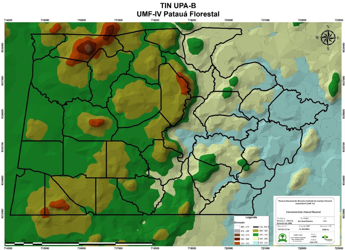
Figura 3. Modelamento TIN, UPA-B, UMF IV, Pataú, Altamira/PA.
