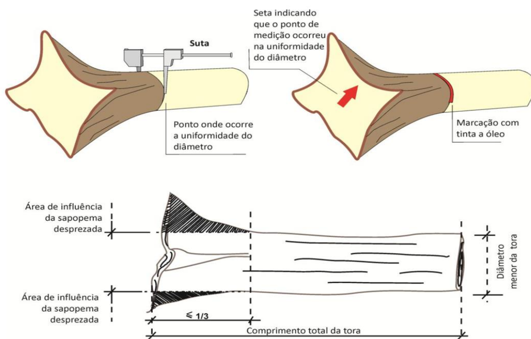
Figura 31: Ponto de medição dos diâmetros em toras com sapopema de até \frac{1}{3} da extensão da tora 3 .
