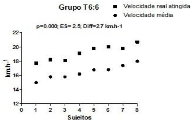
Figura 7 - Diferença entre velocidade média e velocidade real atingida no PV no grupo T6:6.
