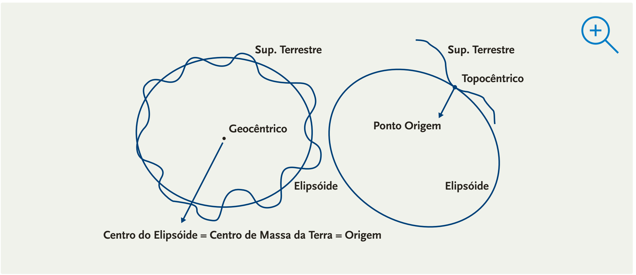
Figura 32 - Origem de um Datum Geodésico Planimétrico Fonte (adaptado): http://www.uff.br/sigcidades/images/Download/sgb_sigcidades_2012.pdf
