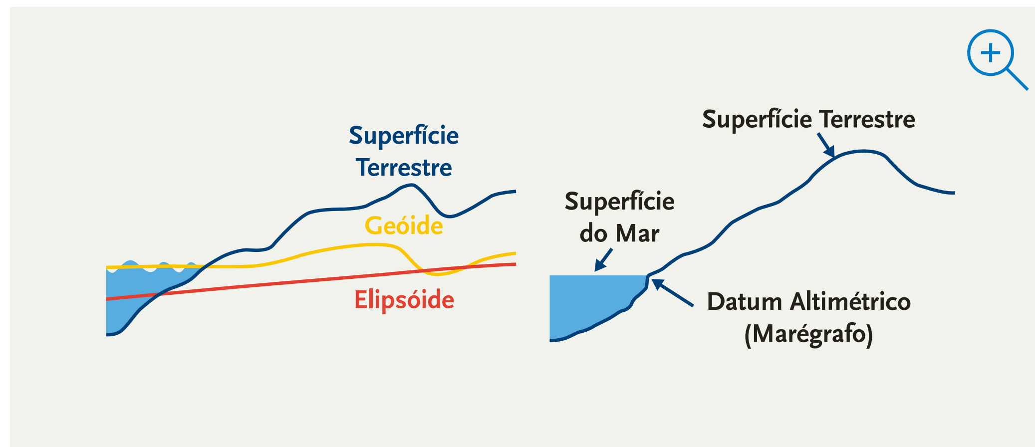
Figura 56 - Geóide e Datum Geodésico Altimétrico
