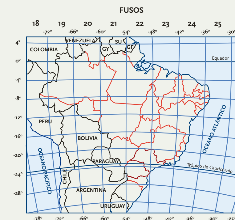
Figura 35 - Fusos da Projeção UTM (Brasil) Fonte (adaptado): http://www.processamentodigital.com.br
