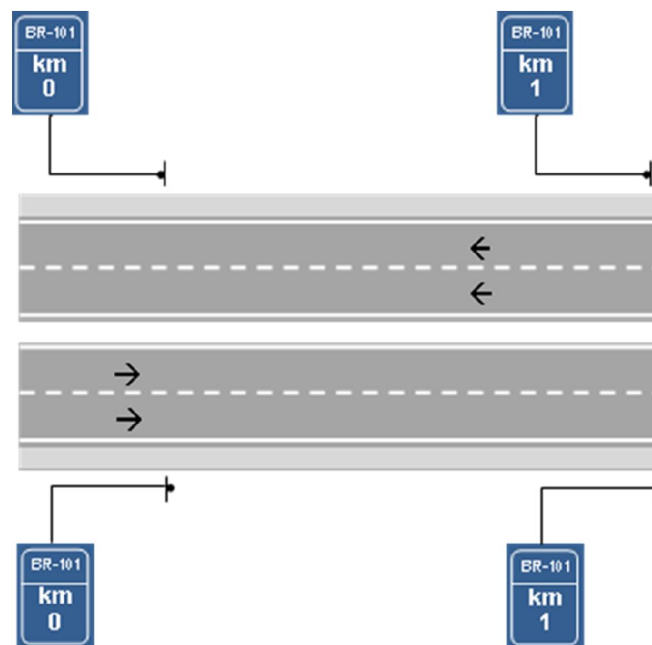
FIGURA 12 - MARCOS QUILOMÉTRICOS EM PISTA DUPLA
