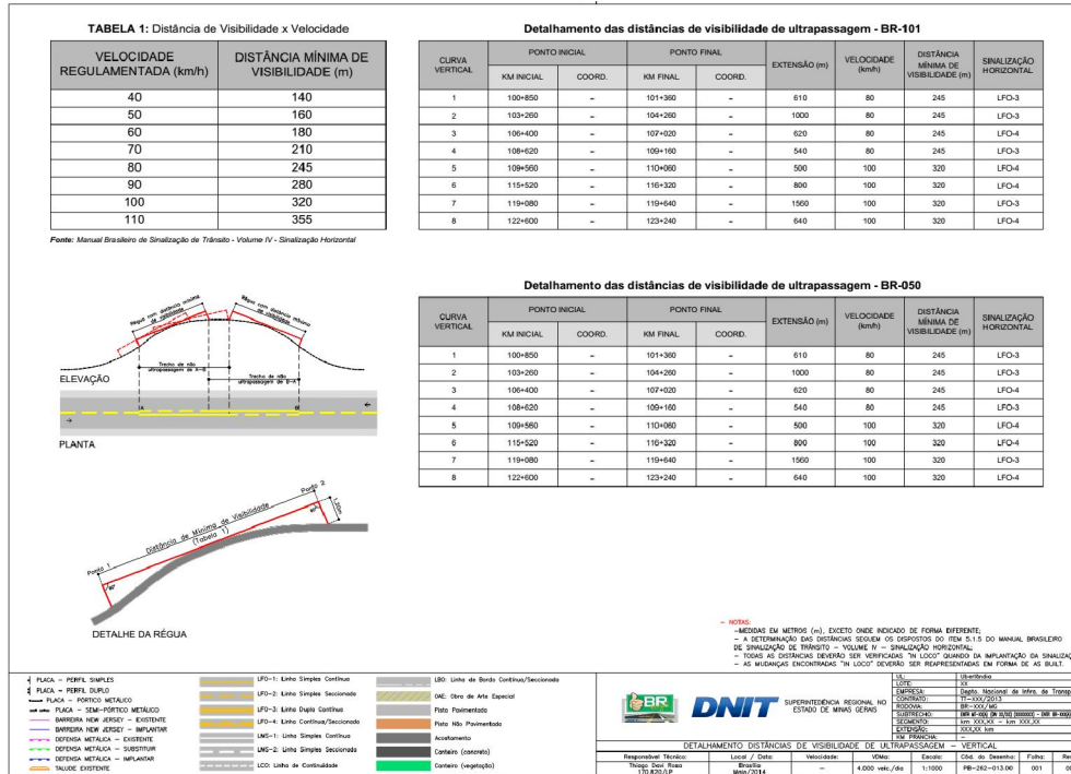
FIGURA 3 - DISTÂNCIA DE VISIBILIDADE DE ULTRAPASSAGEM - VERTICAL
