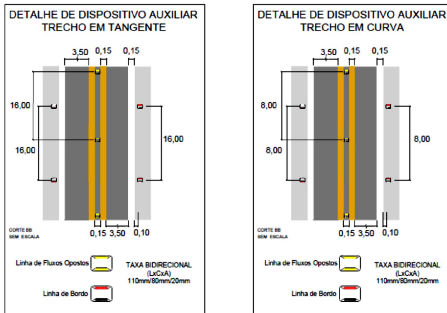
FIGURA 18 - DETALHE DOS DISPOSITIVOS
