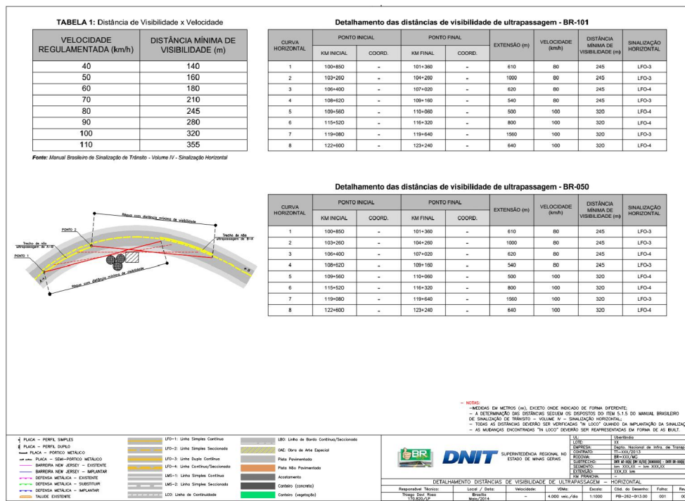
FIGURA 2 - DISTÂNCIA DE VISIBILIDADE DE ULTRAPASSAGEM - HORIZONTAL
