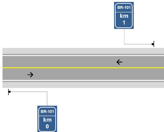
FIGURA 11 - ALTERNÂNCIA DOS MARCOS QUILOMÉTRICOS
