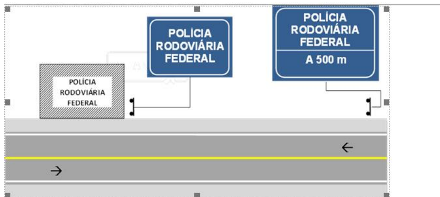
FIGURA 7 - ESQUEMA GERAL DE PRÉ-SINALIZAÇÃO PARA PRF
