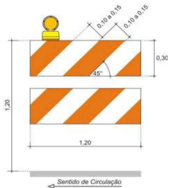
Barreira Tipo II
