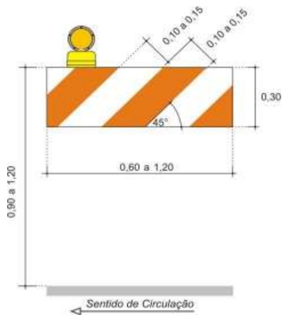
Barreira Tipo I
