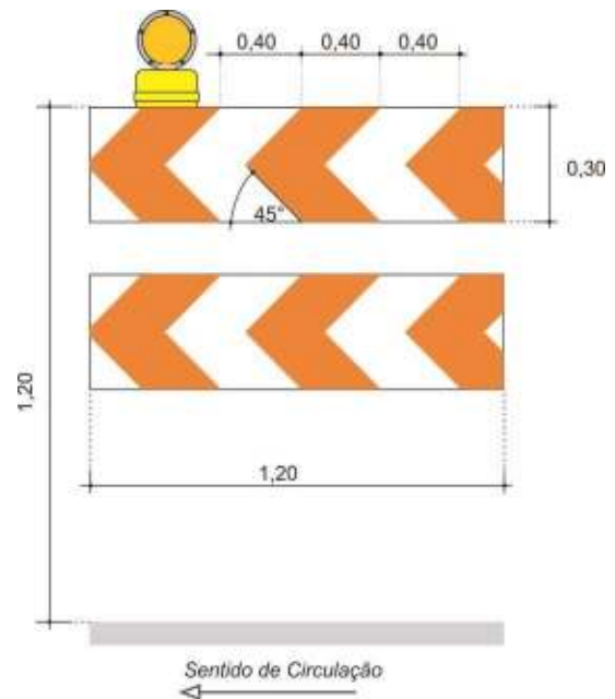
Barreira Tipo II
