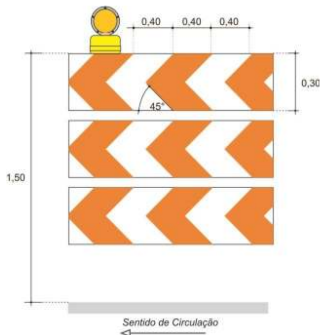
Barreira Tipo III
