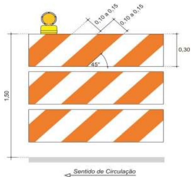
Barreira Tipo III
