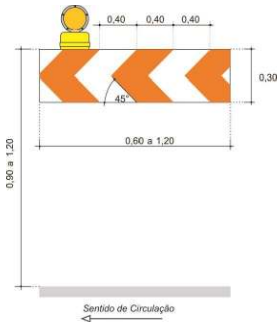
Barreira Tipo I
