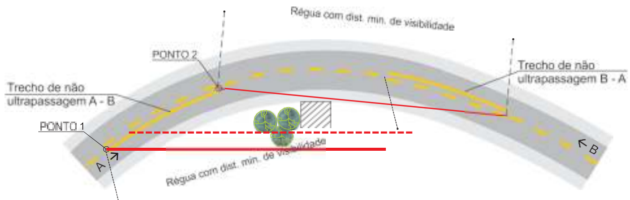
FIGURA 2: Distância de Visibilidade de Ultrapassagem – Horizontal.
