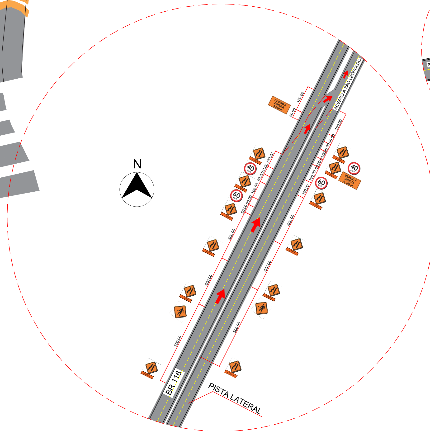
DETALHE 4
