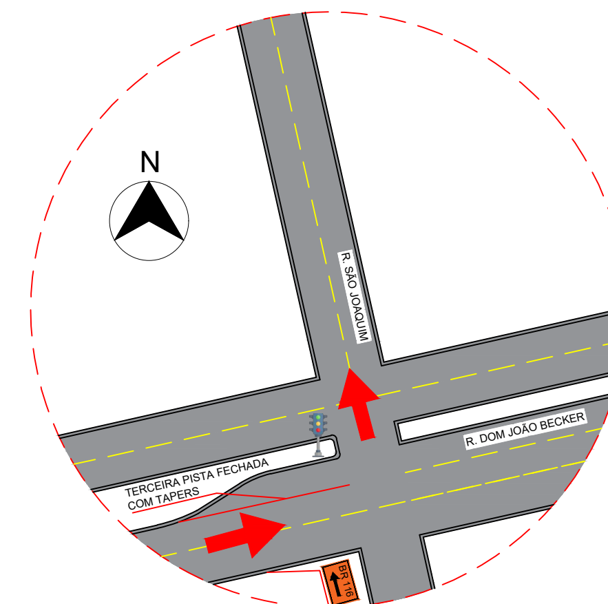
DETALHE 3
