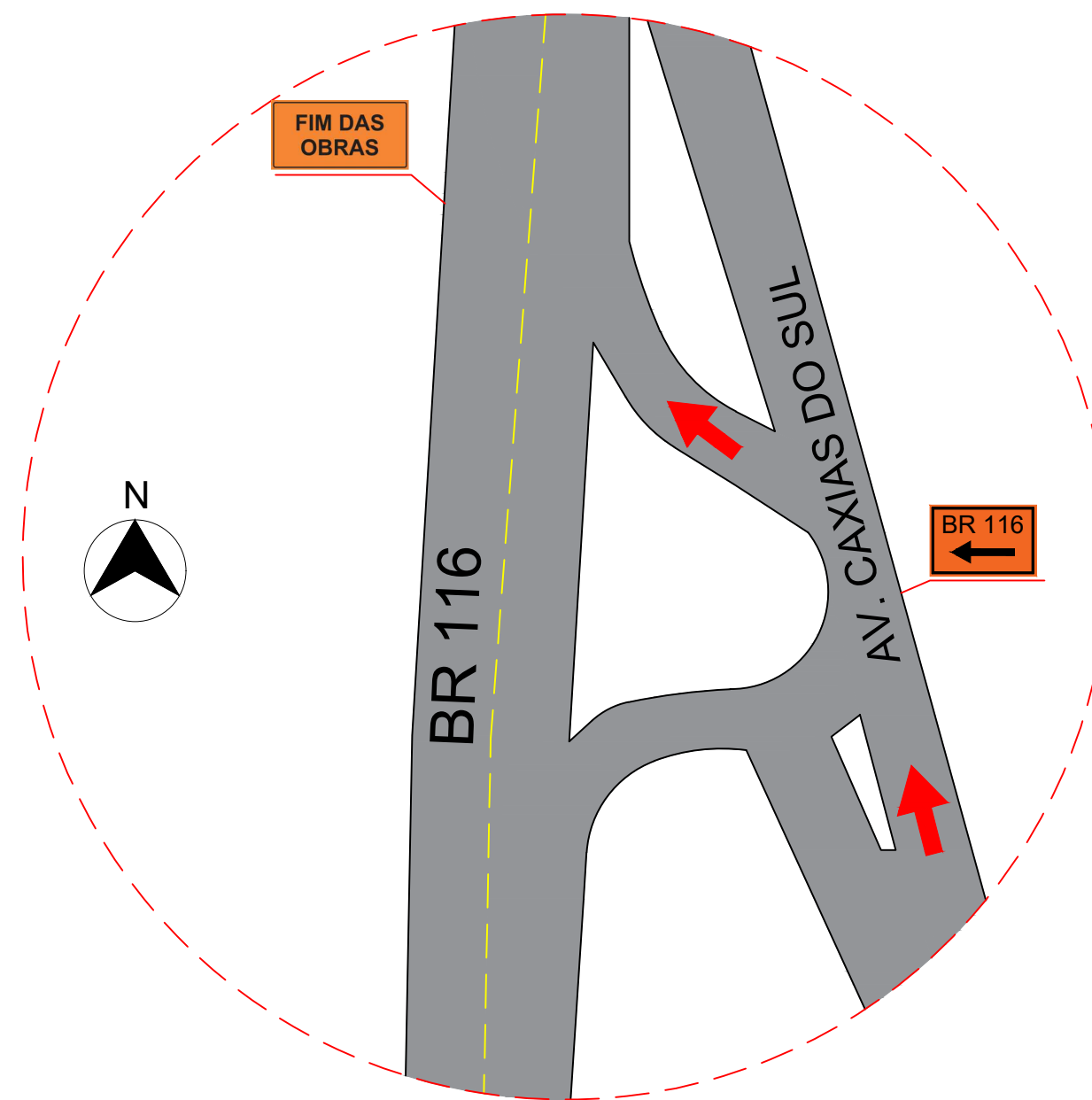
DETALHE 4
