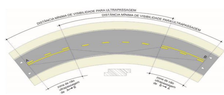
Figura 3: Distância de visibilidade de ultrapassagem horizontal
