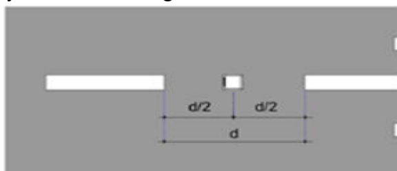
Figura 6: Posição da tacha junto à marca longitudinal seccionada amarela, no eixo da linha simples
