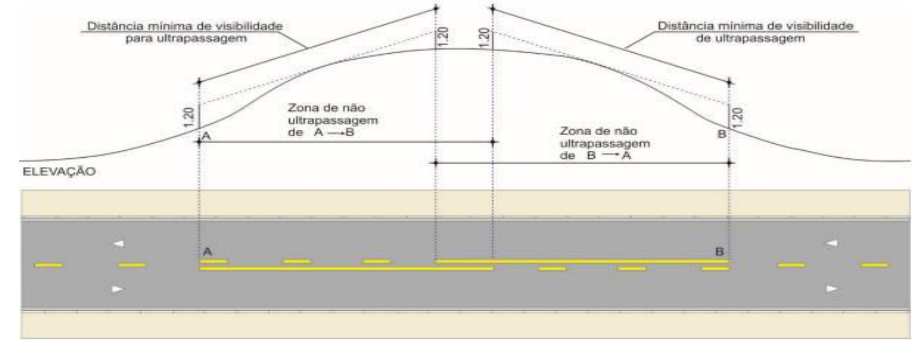
Figura 4: Distância de visibilidade de ultrapassagem vertical
