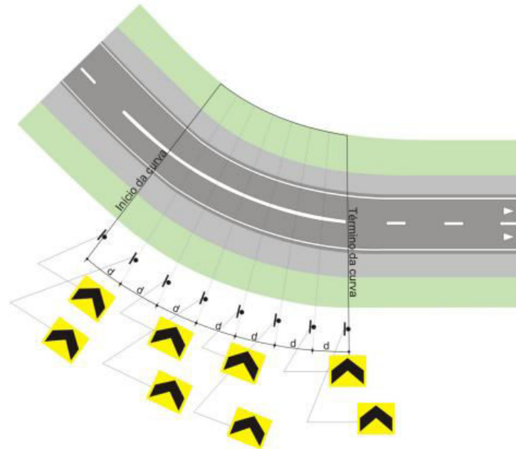
Figura 2: Implantação de marcadores de alinhamento
