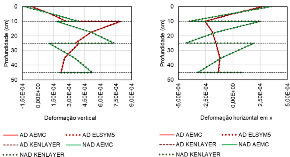
Figura 5 – Deformações verticais e horizontais (aderido AD versus não aderido NAD) (a) Deformação vertical (b) Deformação horizontal
