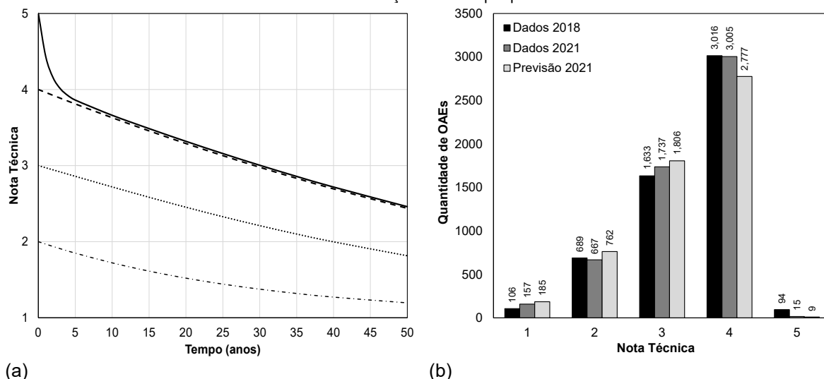
Figura 1 – Saídas do modelo de deterioração para a amostra contendo 6.383 OAEs: (a) Curvas de deterioração; (b) Previsão do estado de condição futuro do parque de obras
