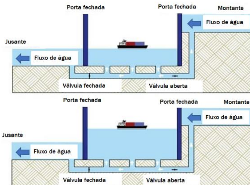
Figura 2 – Processo de enchimento da câmara de eclusagem
