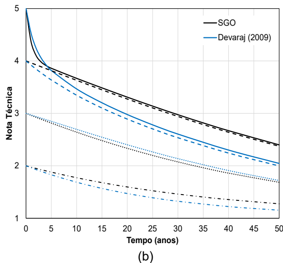
Figura 3 – Curvas de deterioração por grupo de OAEs: (a) OAEs com até 20 anos de idade; (b) OAEs com idade entre 20 e 40 anos; (c) OAEs com 41 ou mais anos de idade
