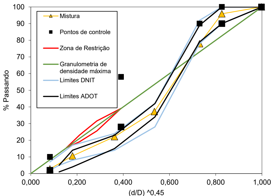
Figura 1 – Curva granulométrica adotada, limites máximo e mínimo segundo a faixa do DNIT, plotados juntamente com a curva de densidade máxima, pontos de controle e zona de restrição para o TNM de 12,5mm
