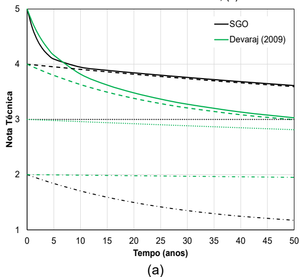
Figura 3 – Curvas de deterioração por grupo de OAEs: (a) OAEs com até 20 anos de idade; (b) OAEs com idade entre 20 e 40 anos; (c) OAEs com 41 ou mais anos de idade
