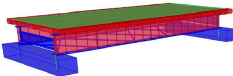
Figura 2.4 – Tabuleiro misto
