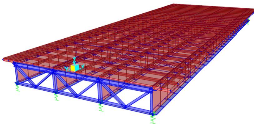
Figura 2.5 – Modelo numérico de pontes mistas
