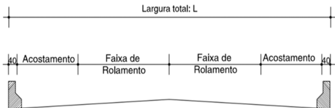
Figura 2.1 – Tipologia da ponte com pista simples
