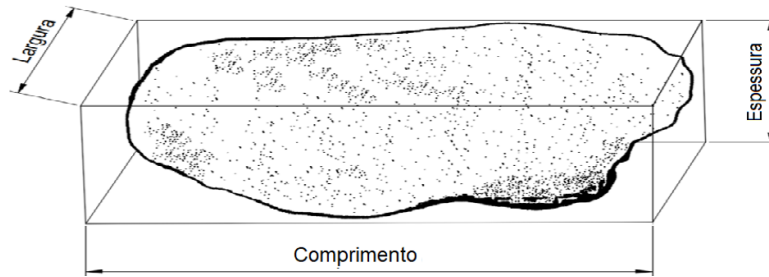
Figura A1 – Definição das dimensões de uma partícula de agregado graúdo.
