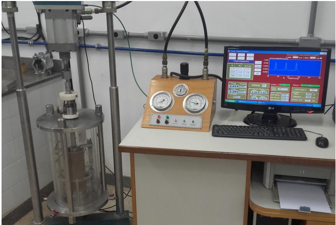
Foto - Exemplo de Equipamento triaxial com LVDTs fixados no cabeçote superior e apoiados em hastes guias.
