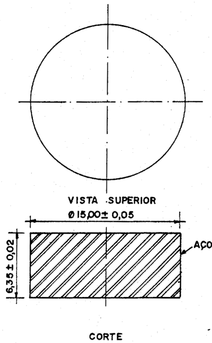
FIGURA 2 - DISCO ESPAÇADOR
