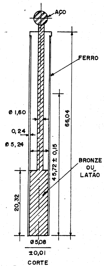
FIGURA 3 - SOQUETE
