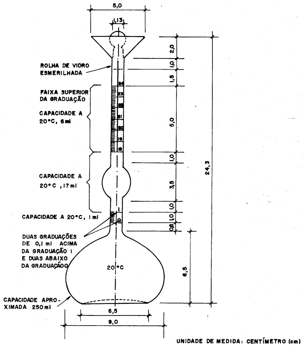
FIGURA I - FRASCO DE LE CHATELIER
