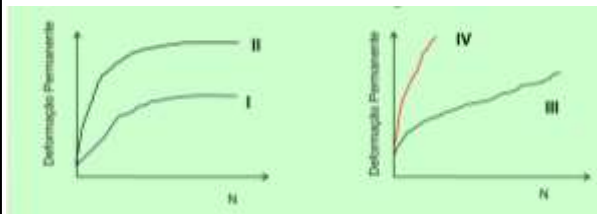
Figura 1 – Modelos de comportamento à deformação permanente de vários materiais ou de um mesmo material a vários níveis de sollicitação de carga cíclica.
