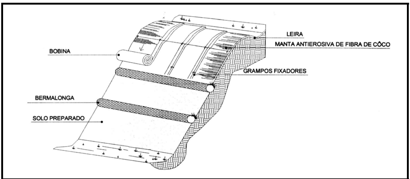
Figura 3 – Esquema representativo da instalação das telas e mantas biodegradáveis, mostrando a aplicação e fixação
