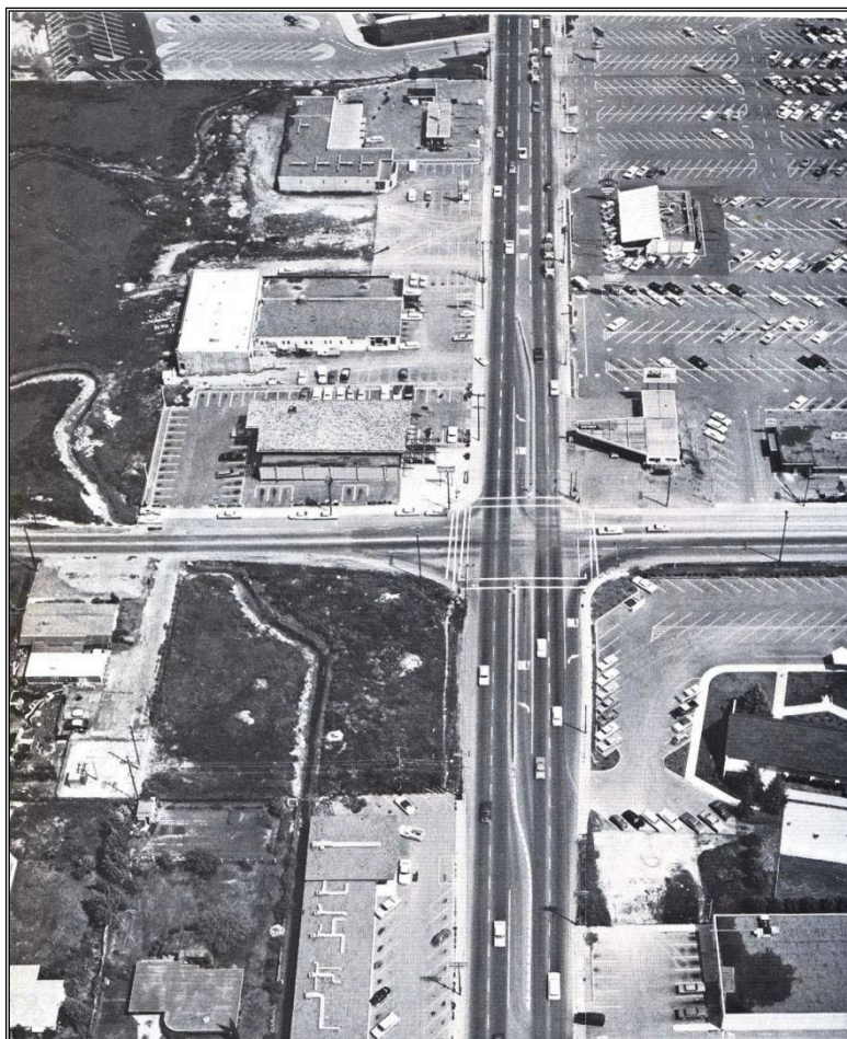
Figura 87 – Faixas de giro à esquerda atendendo os dois sentidos do tráfego
