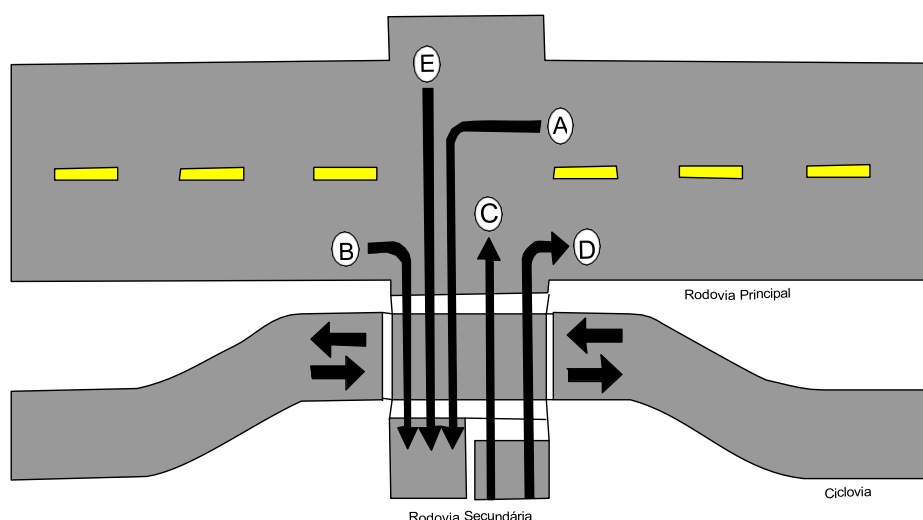
Figura 28 – Interseção de ciclovias adjacente à rodovia
