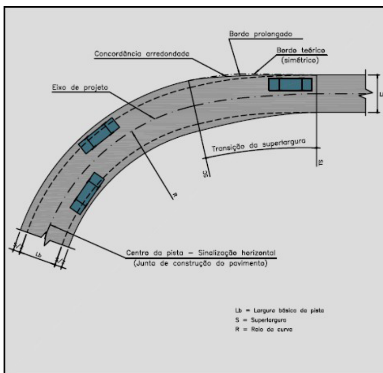
Figura 73 – Exemplo de superlargura obtida por alargamento simétrico da pista
