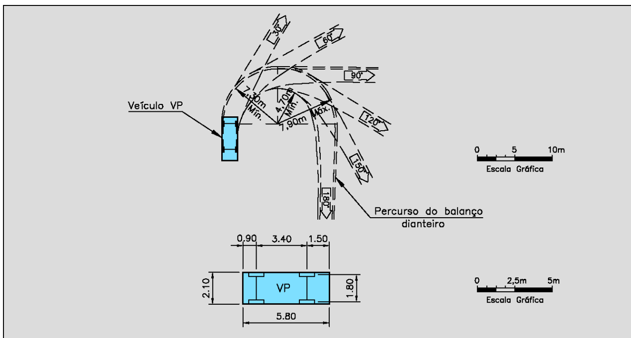
Figura 46 – Veículo de Projeto VP
