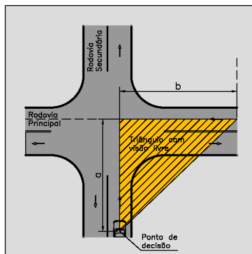
Figura 61 – Triângulo de visibilidade para o veículo em movimento (Dê a Preferência)
