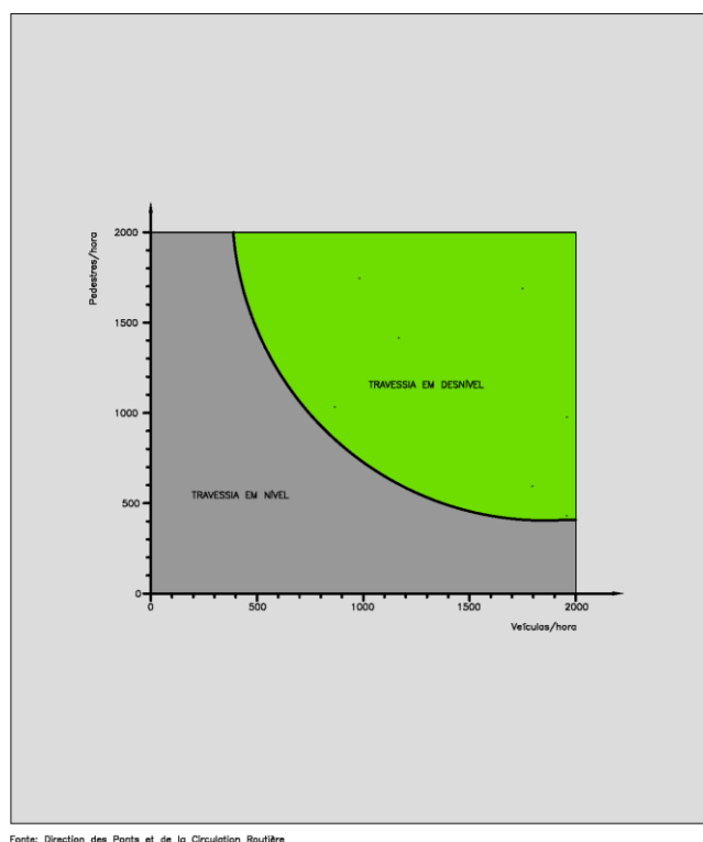
Figura 15 – Fluxos que justificam a implantação de passarelas
