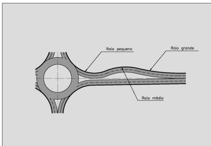
Figura 108 – Curvas sucessivas nas aproximações das rótulas em vias rurais de alta velocidade
