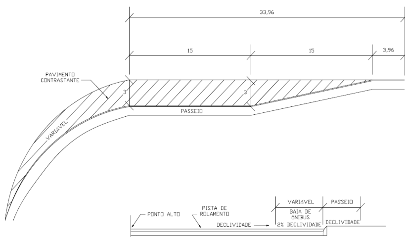
Figura 36 – Baia de ônibus depois da esquina
