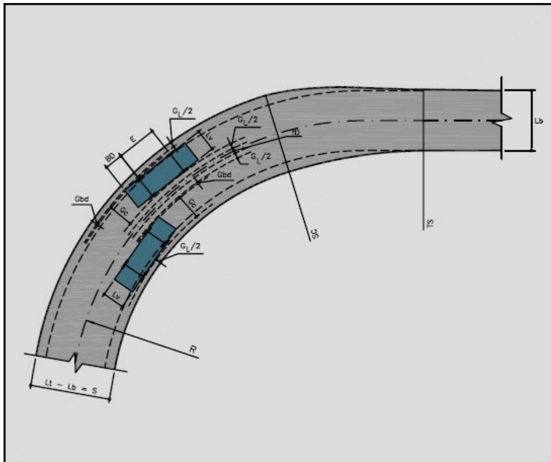
Figura 72 – Elementos intervenientes no cálculo da superlargura
