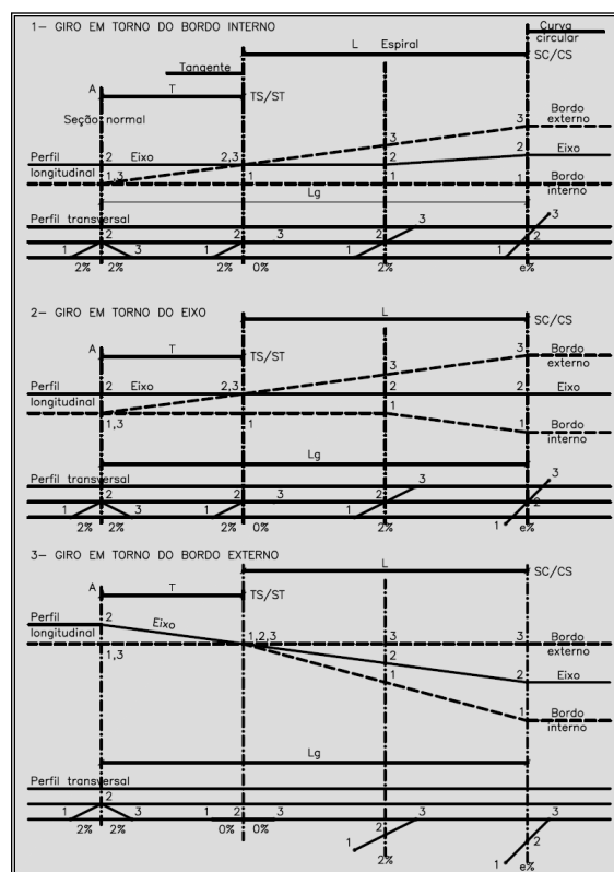
Figura 70 – Métodos de giro de acordo com a posição do eixo de rotação (Declividade transversal em dois sentidos)
