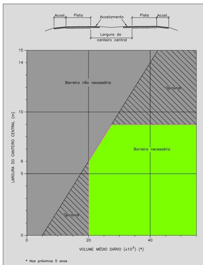
Figura 92 – Necessidade de defesa ou barreira rígida em canteiros centrais
