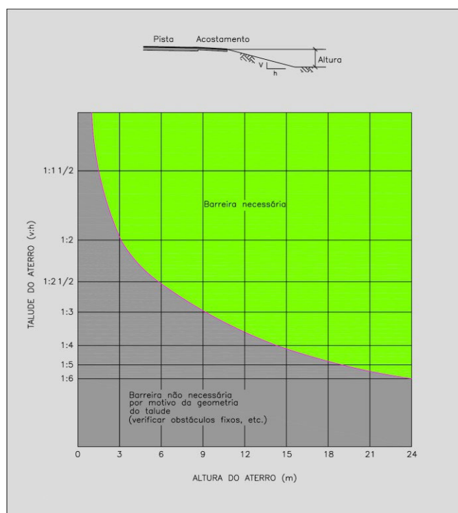
Figura 91 – Necessidade de defesa ou barreira rígida em aterros
