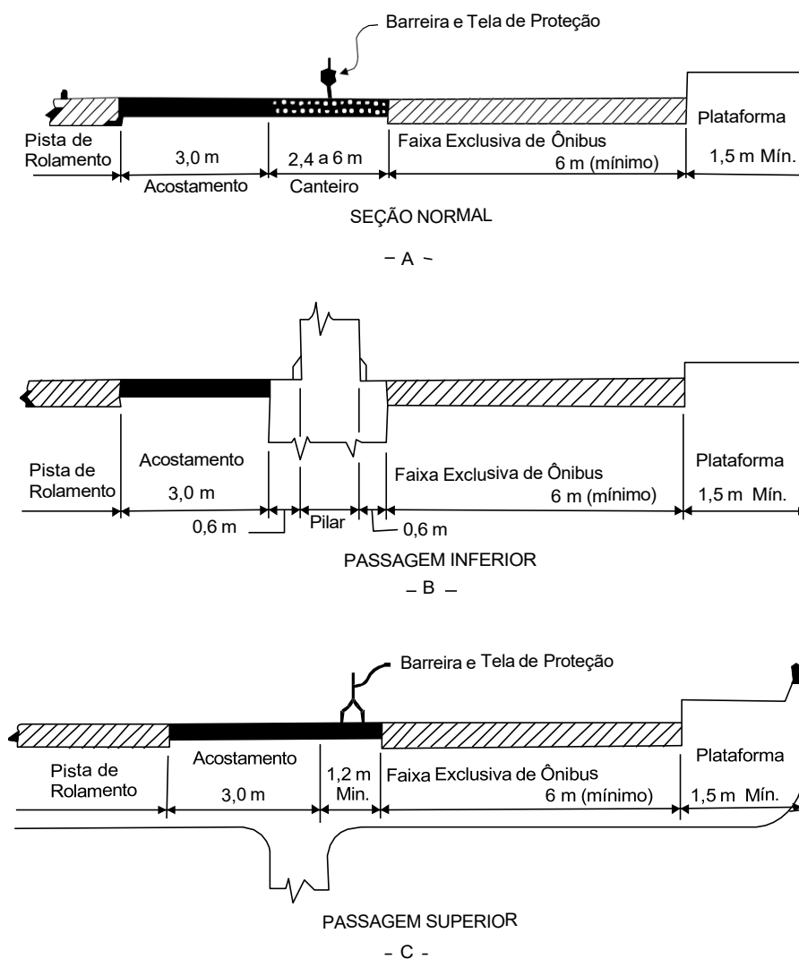
Figura 35 – Seções transversais típicas de baias de ônibus nas vias expressas
