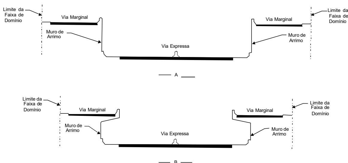
Figura 99 – Seções transversais com muros de arrimo
