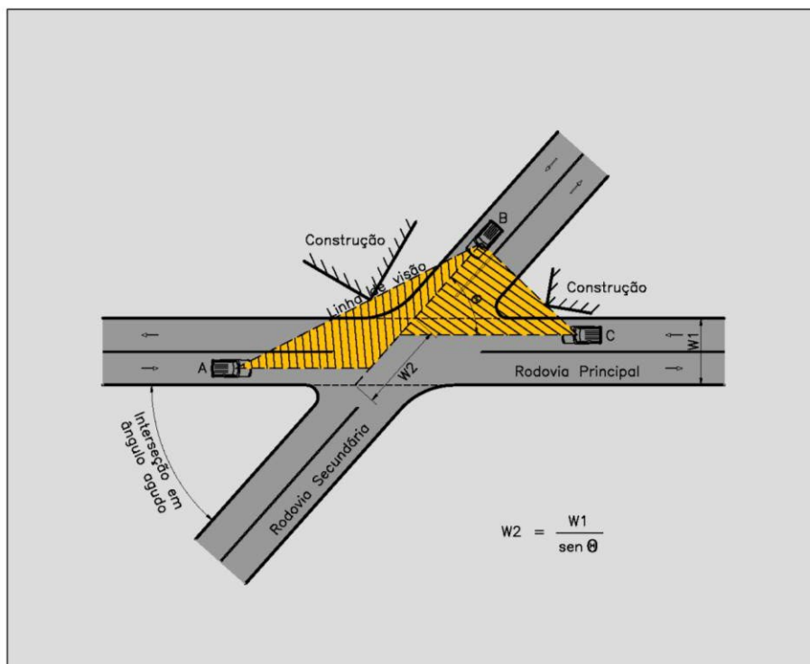
Figura 63 – Triângulo de visibilidade em interseções esconsas
