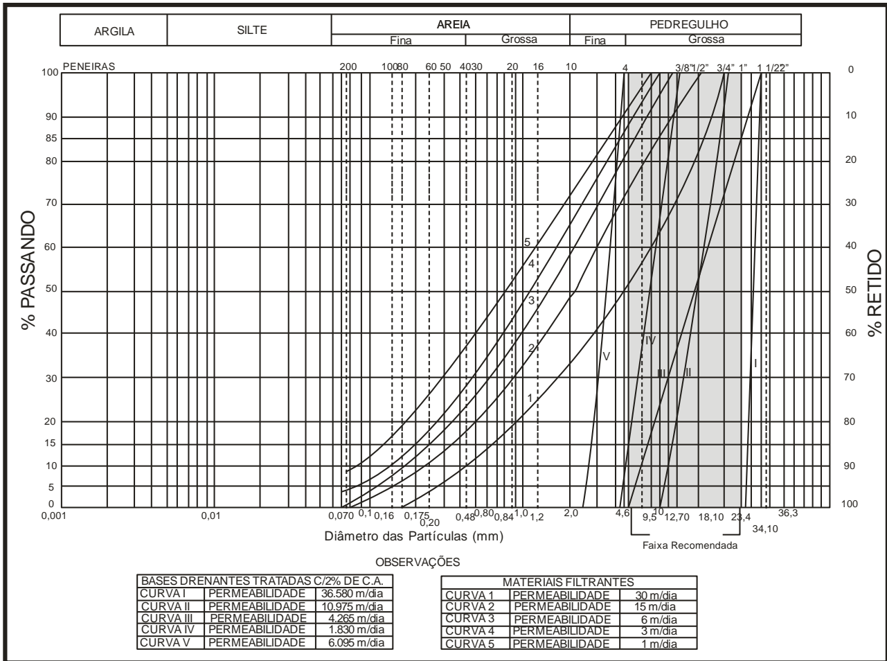
Figura 54 - Curvas granulométricas
