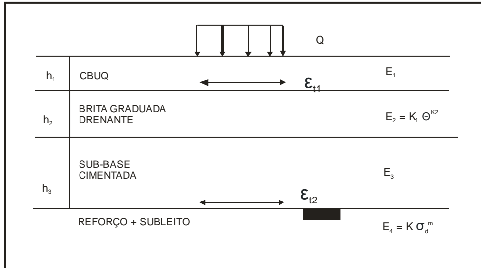
Figura 47 - Pavimento invertido
