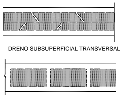
Figura 53 - Alguns tipos de drenos utilizados em projetos de rodovias
