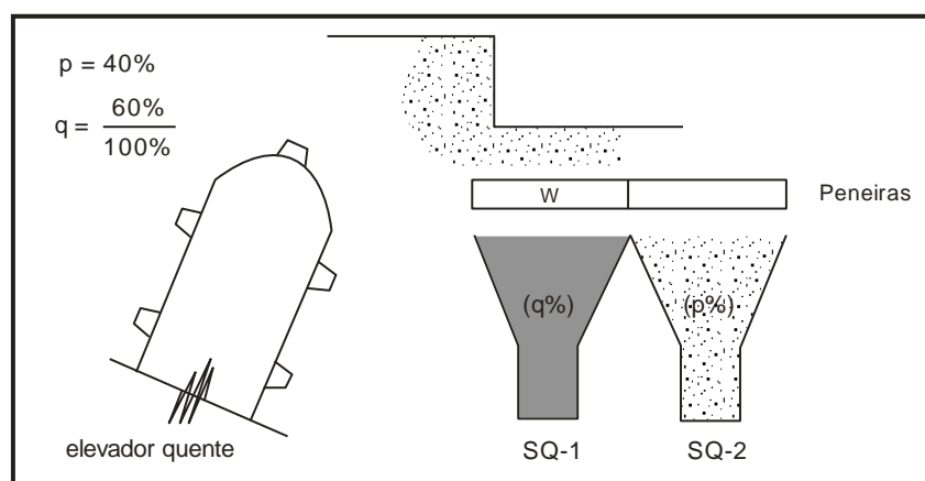
Figura 64 - Agregado do secador para os silos quentes
