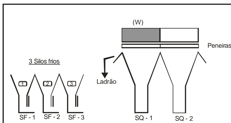
Figura 63 - Usina com 3 silos frios e 2 silos quentes
