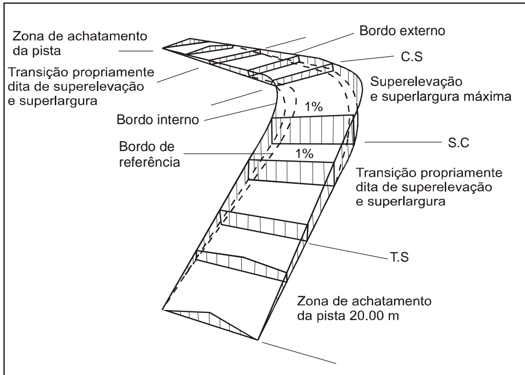
Figura 32 - Superelevação
