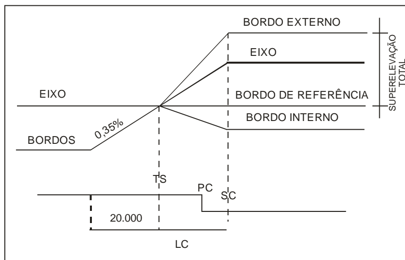
Figura 33 - Esquema de superelevação
