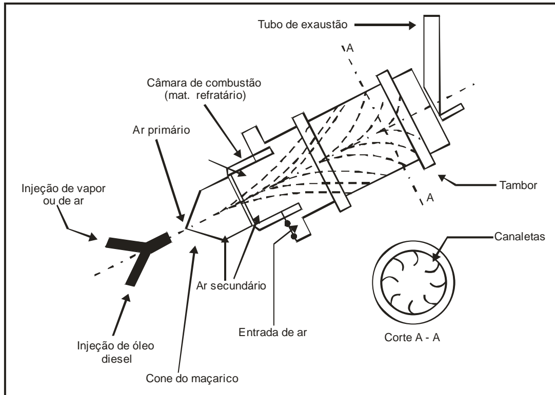
Figura 62 - SECADOR - corte A - A
