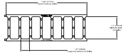
VISTA SUPERIOR - Grelha
