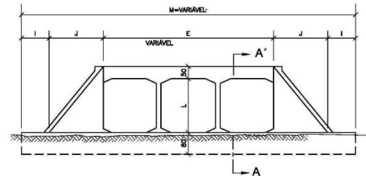
VISTA EM ELEVACÃO
