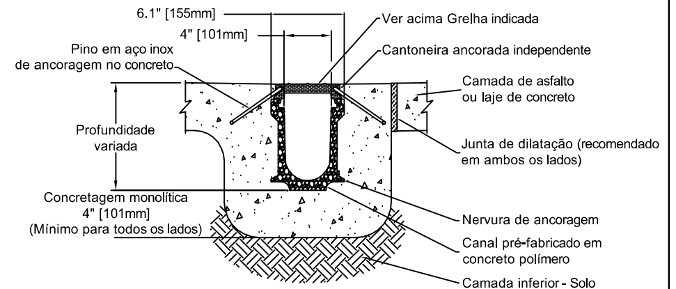
SEÇÃO TRANSVERSAL
