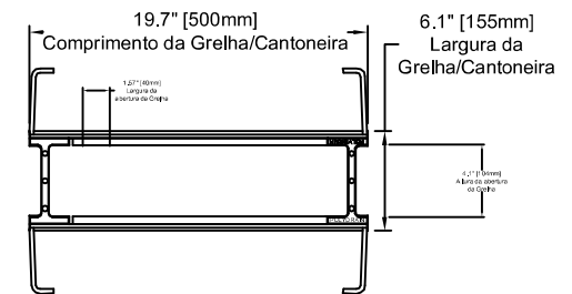
VISTA SUPERIOR - Grelha e Cantoneira
