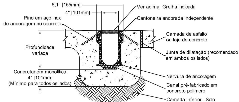
SEÇÃO TRANSVERSAL
