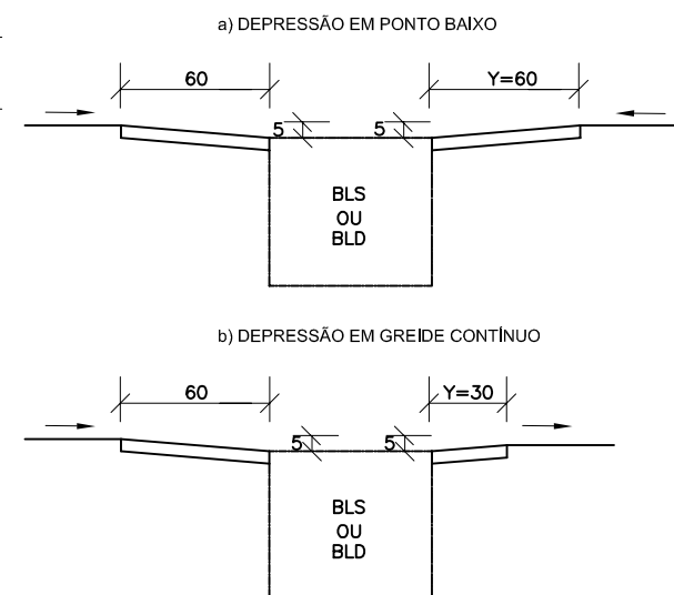
CORTE LONGITUDINAL
