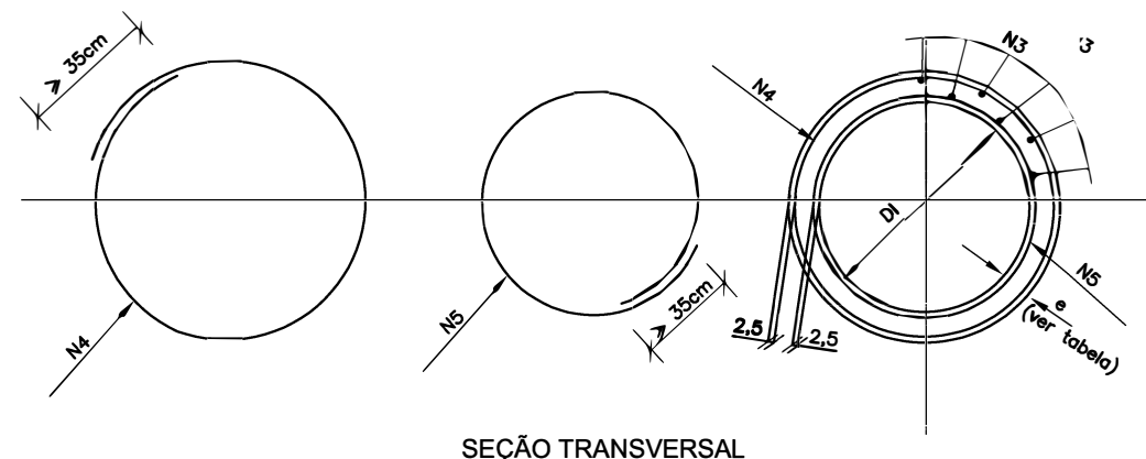
SEÇÃO TRANSVERSAL
