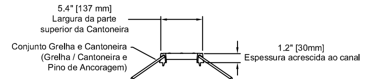
VISTA FRONTAL - Grelha e Cantoneira
