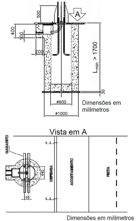
Detalhe 1 - Esboço da base de suporte do semipórtico metálico
