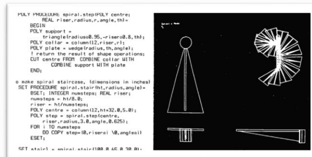
GLIDE (primeiro software de design paramétrico)
