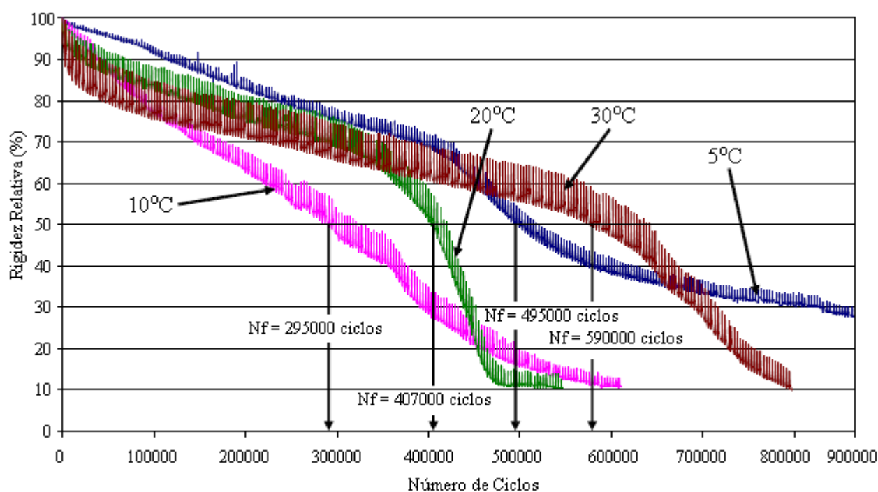
Figura 3 - Curvas de fadiga para diferentes temperaturas (DOMEC, 2005).
