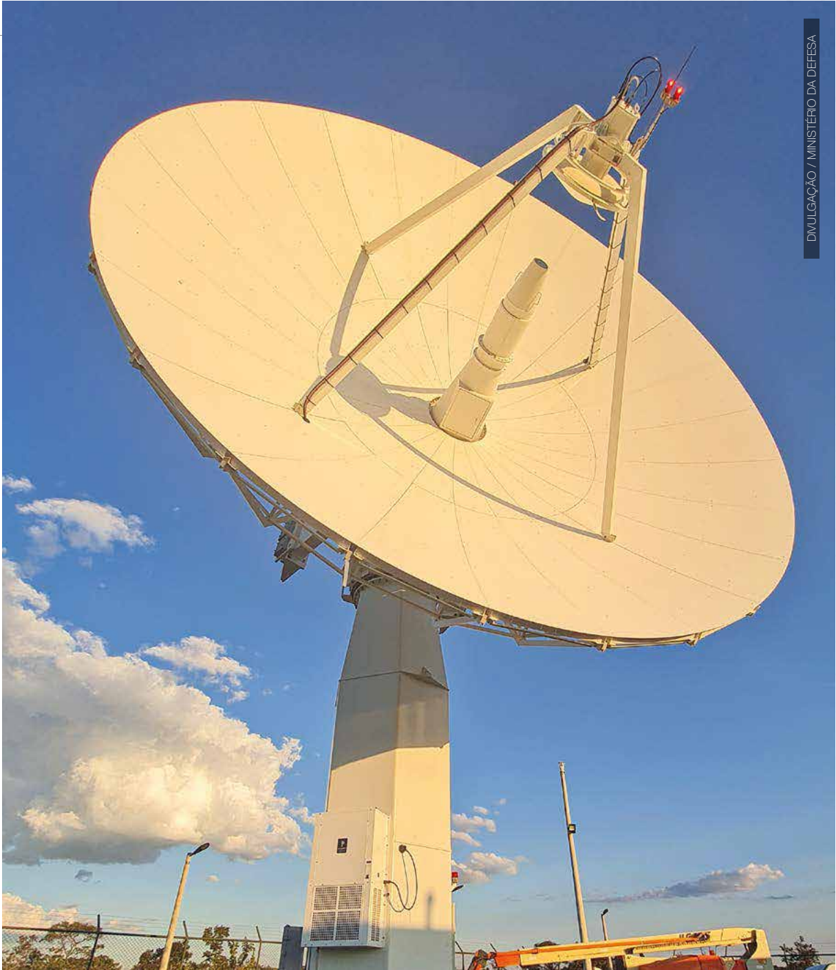
Antena multisatelital de observação da Terra
