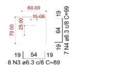
S6=S8=S12=S13=S23=S28 PLANTA ESC 1:25
