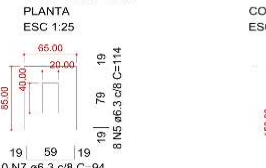
S17=S18=S19 PLANTA ESC 1:25
