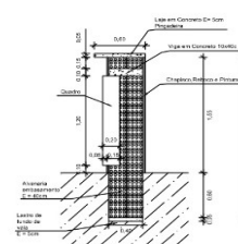
Detalhe da Mureta
