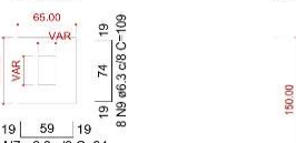
S32=S34=S35=S36=S38 PLANTA ESC 1:25
