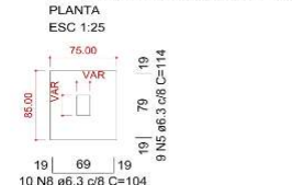
S1=S3=S4=S5=S9=S21=S22=S26=S30 PLANTA ESC 1:25
