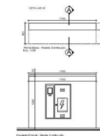
Detalhe da Mureta
