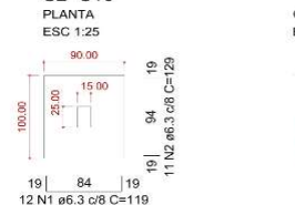
S2=S10 PLANTA ESC 1:25
