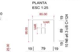
S11=S14=S15=S24=S25=S29=S37 PLANTA ESC 1:25
