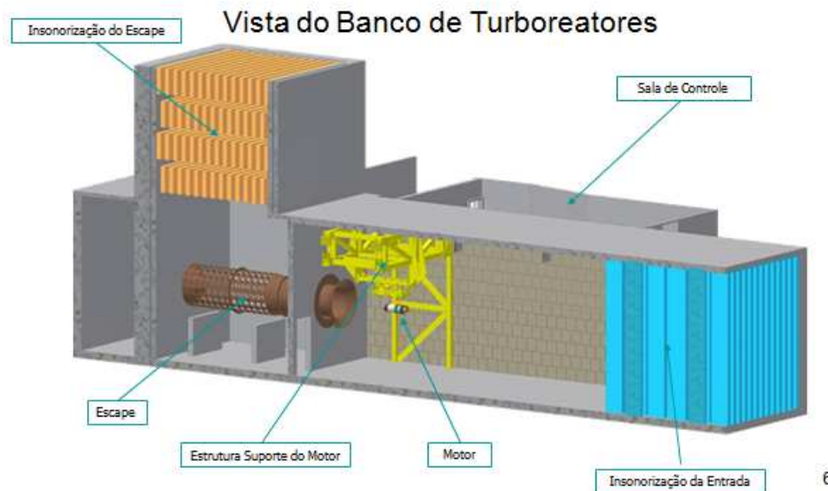
Imagem com o layout da sala de ensaios.
