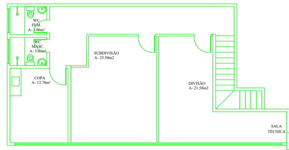
PLANTA BAIXA - 1º PAV. PLANTA DE MODIFICAÇÃO ESC: 1/75 LEGENDA: - DEMOLIR = CONSTRUIR = MANTER
