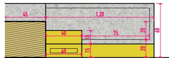
Arquibancadas 1:25
