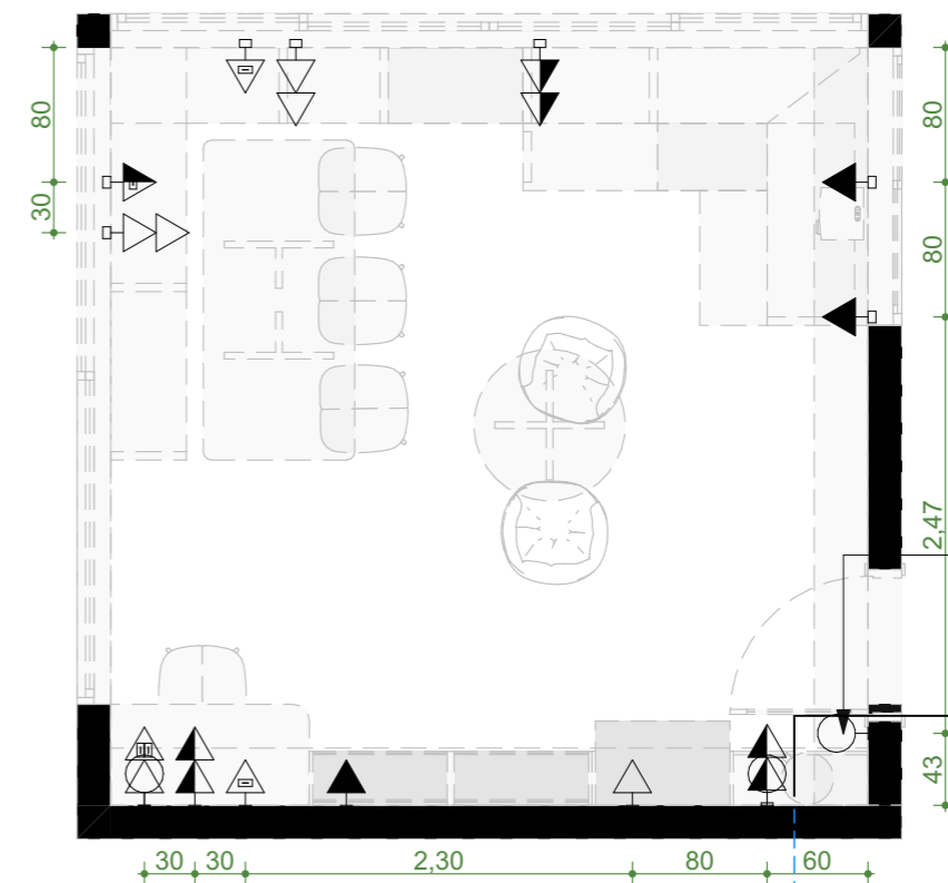
1:50 Elétrica Básica
