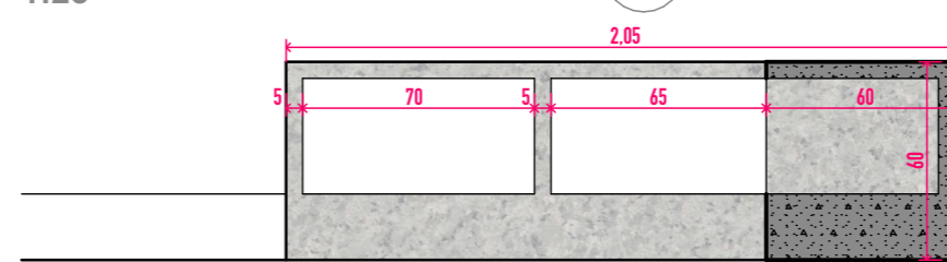
Arquibancadas - visão livre 1:25
