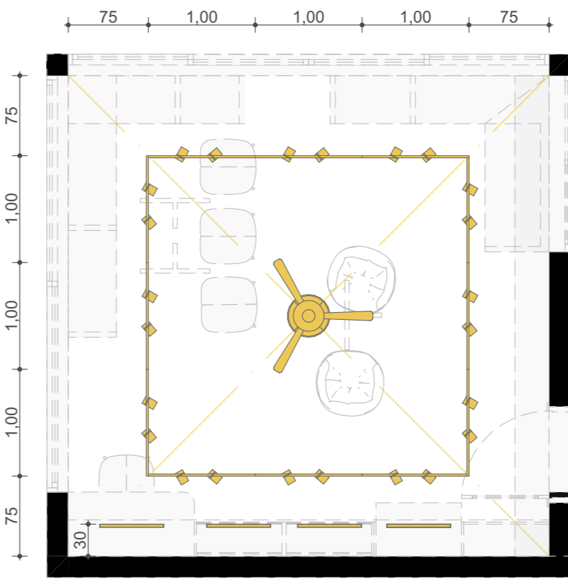
1:50 Iluminação
