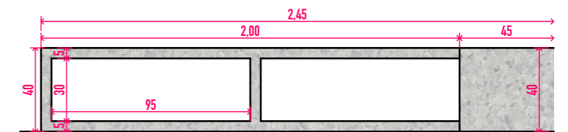
Banco da Mesa Coletiva 1:25
