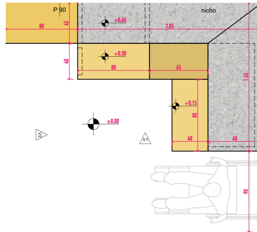
Arquibancadas - Vista de topo 1:25
