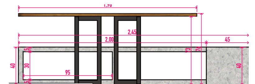
Mesa Coletiva 1:25
