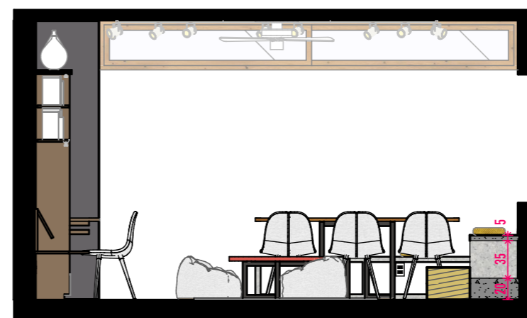
Corte
