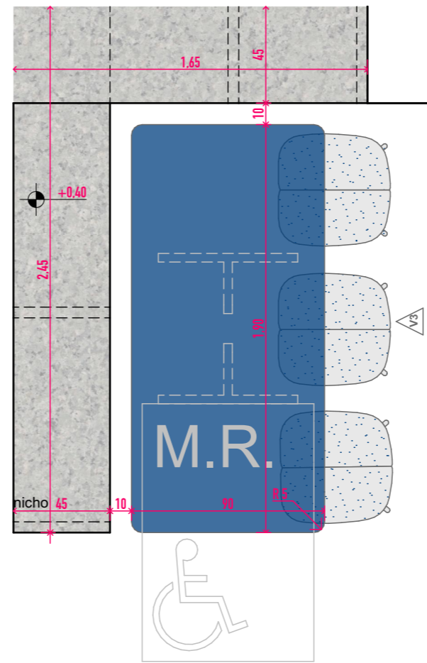
Arquibancadas - Vista de topo 1:25
