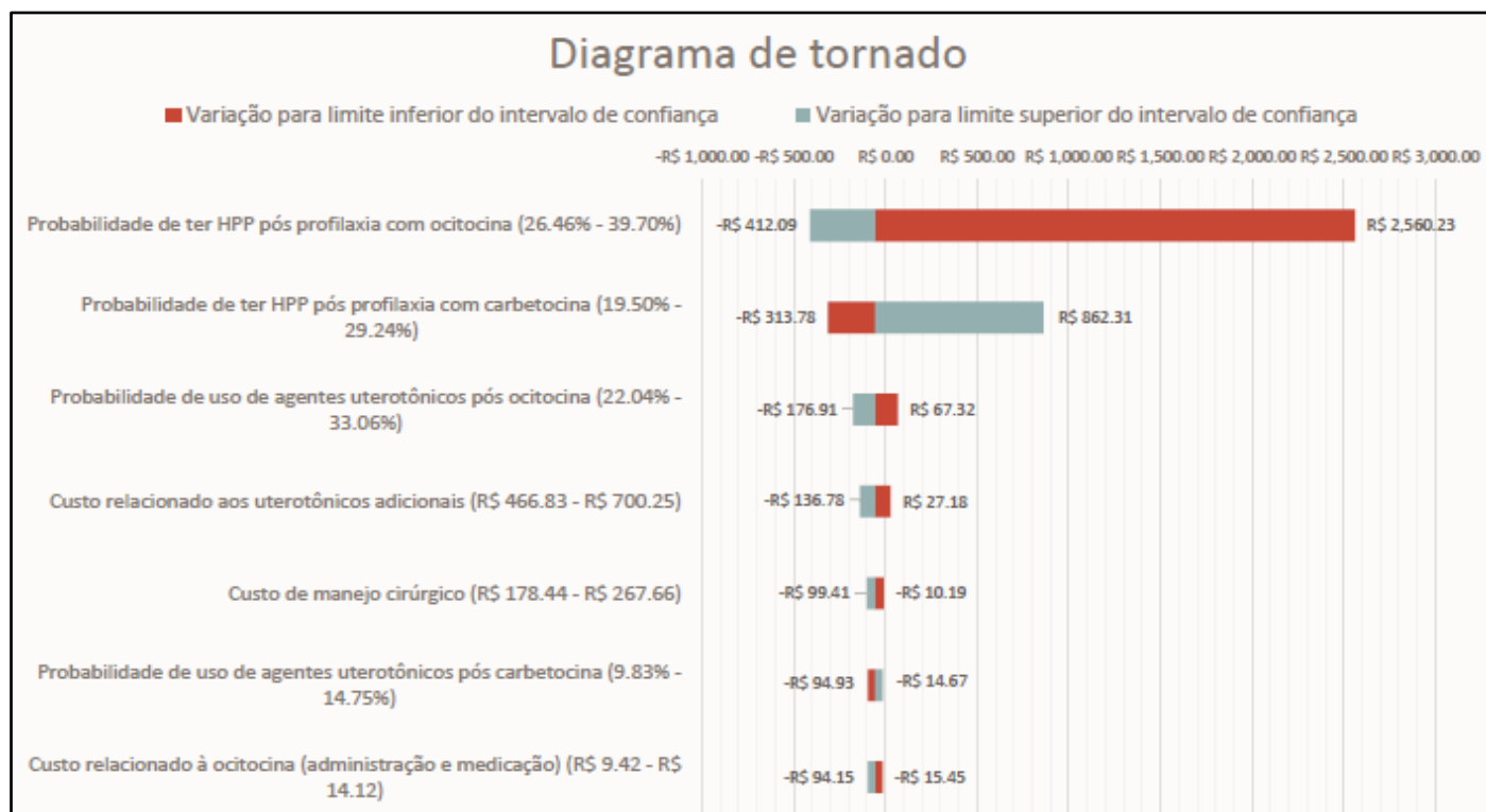
Figura 22. Diagrama de tornado – taxa de desperdício
