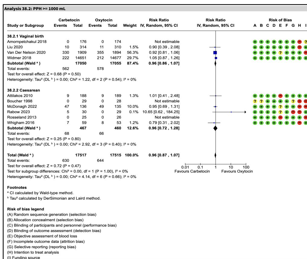
Figura 16. Metanálise desfecho HPP \geq 1000ml
