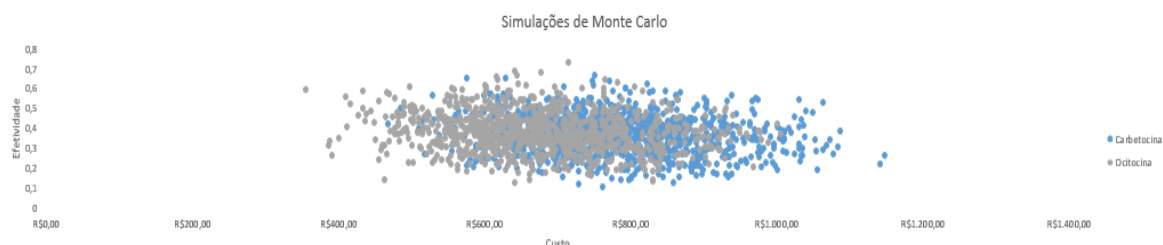
Figura 8. Simulação Monte Carlo sem taxa de desperdício – parecerista
