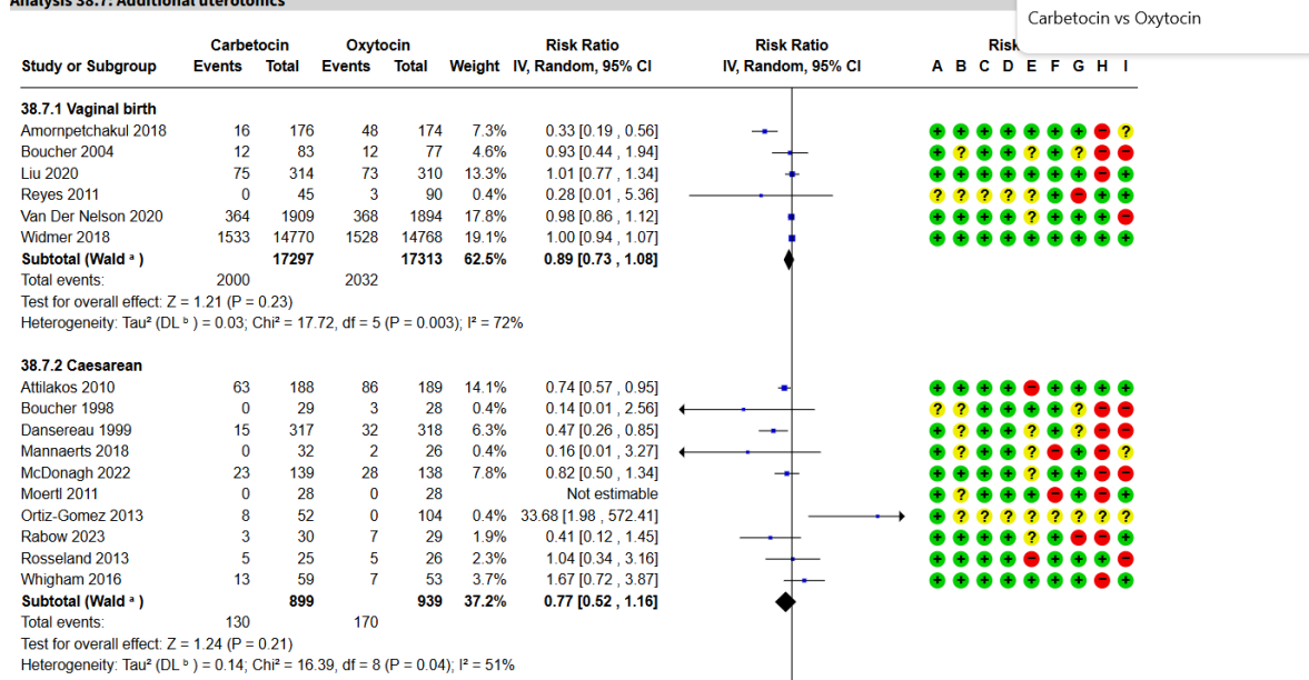
Figura 21. Metanálise desfecho uterotônico adicional.
