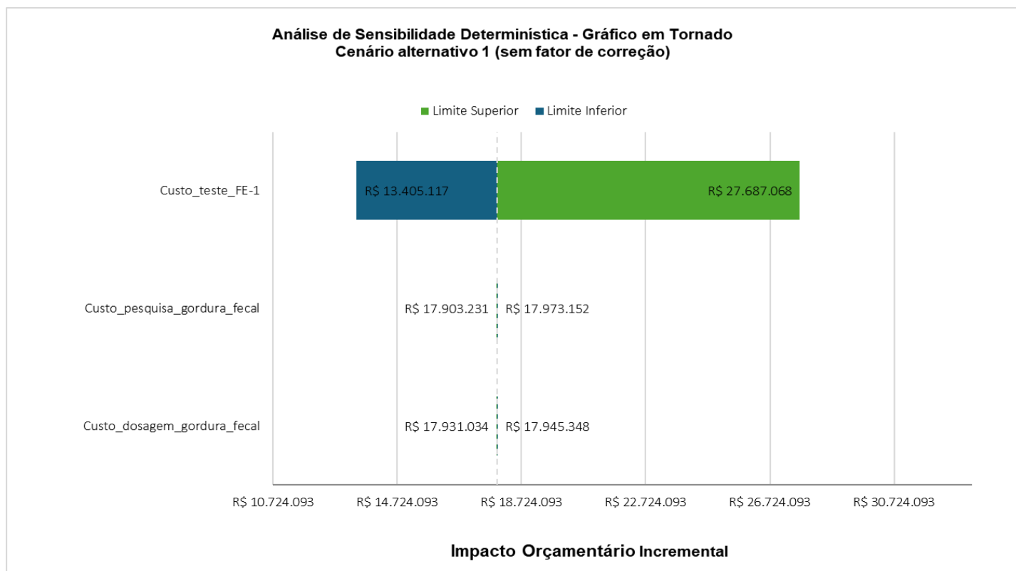
Figura 28. Análise de sensibilidade determinística do tipo gráfico em tornado para o valor acumulado em cinco anos para o cenário alternativo 1 (sem fator de correção).
