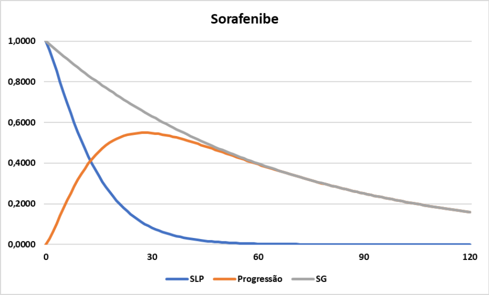
Figura A4. Curvas de extrapolação para sorafenibe
