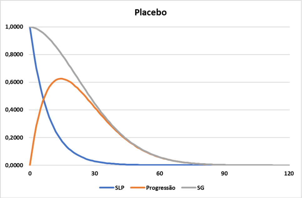
Figura A7. Curvas de extrapolação para placebo
