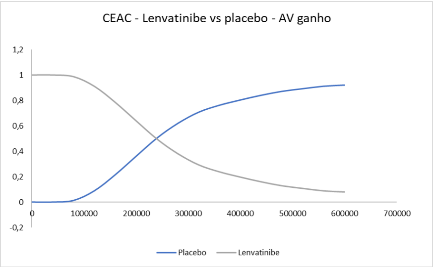
Figura A19. Curva de aceitabilidade (desfecho: anos de vida ganho– Lenvatinibe vs Melhor tratamento de suporte ).
