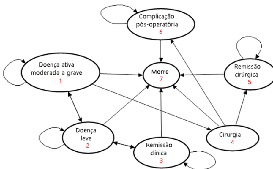
Figura 14. Estrutura do modelo de Markov para a fase de indução com os estados de transição.
