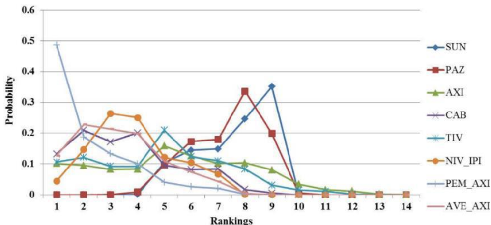
Figura 12 - Classificação dos tratamentos para sobrevida livre de progressão em pacientes de risco intermediário. Legenda: AVE_AXI: avelumabe/axitinibe; AXI: axitinibe; CAB: Cabozantinibe; NIV_IPI: nivolumabe/ipilimumabe; PAZ: pazopanibe; PEM_AXI: pembrolizumabe/axitinibe;; SUN: sunitinibe; TIV: tivozanibe.
