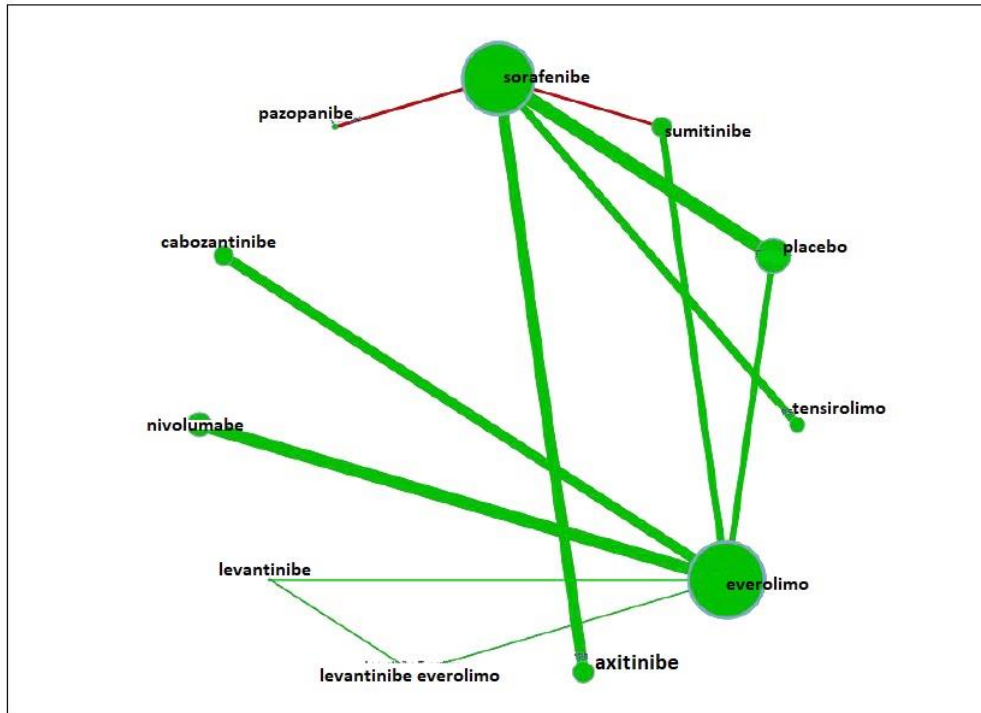
Figura 21 - Network Plot da NMA para taxa de resposta parcial.
