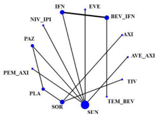
Figura 7 - Diagrama de rede: o tamanho de cada nó de tratamento corresponde ao número de pacientes. Nota: A largura das linhas é proporcional ao número de tentativas. Legenda: AXI: axitinibe; BEV_IFN: bevacizumabe/interferon; EVE: everolimo; IFN: IFN- \alpha ; NIV_IPI: nivolumabe/ipilimumabe; PAZ: pazopanibe; PEM_AXI: pembrolizumabe/axitinibe; PLA: placebo; SOR: sorafenibe; SUN: sunitinibe; TEM_BEV: temsirolimo mais bevacizumabe; TIV: tivozanibe.
