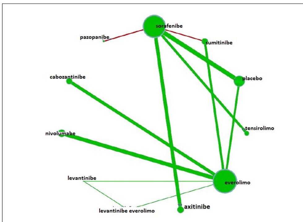
Figura 22 - Network Plot da NMA para taxa de resposta para doença estável.
