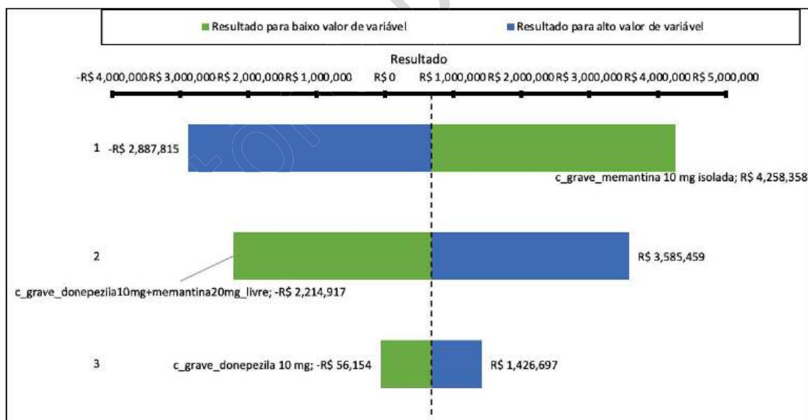
Figura A 11. Gráfico das análise de sensibilidade determinística do impacto orçamentário.
