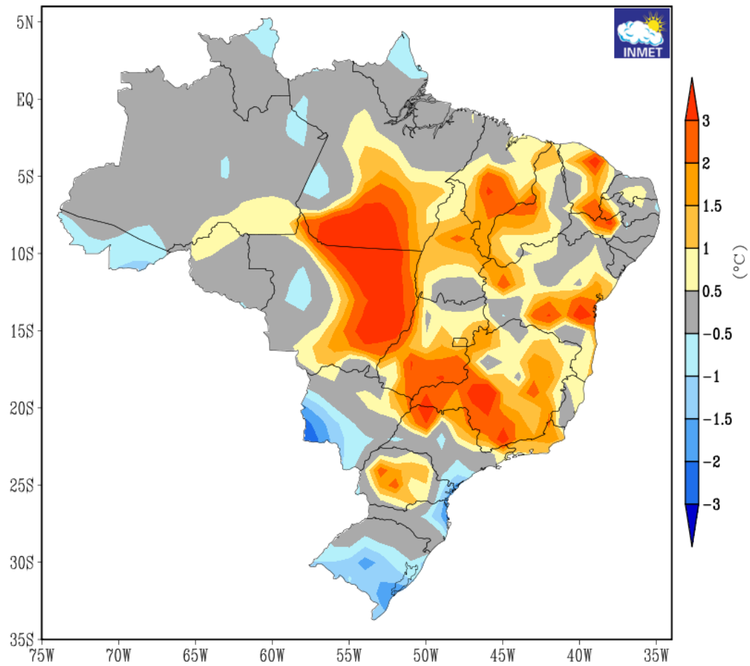
ANOMALIAS DE TEMPERATURAS MÉDIAS VALIDO MAIO de 2026 CLIMATOLOGIA DE REFERÊNCIA: 1991-2020
