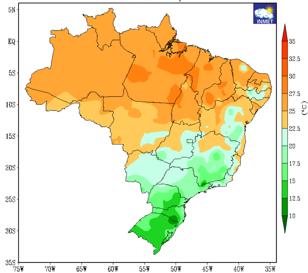
TEMPERATURA MÉDIA PREVISTA (°C) ATUALIZAÇÃO - MAIO/2026 VALIDO PARA JUNHO/2026
