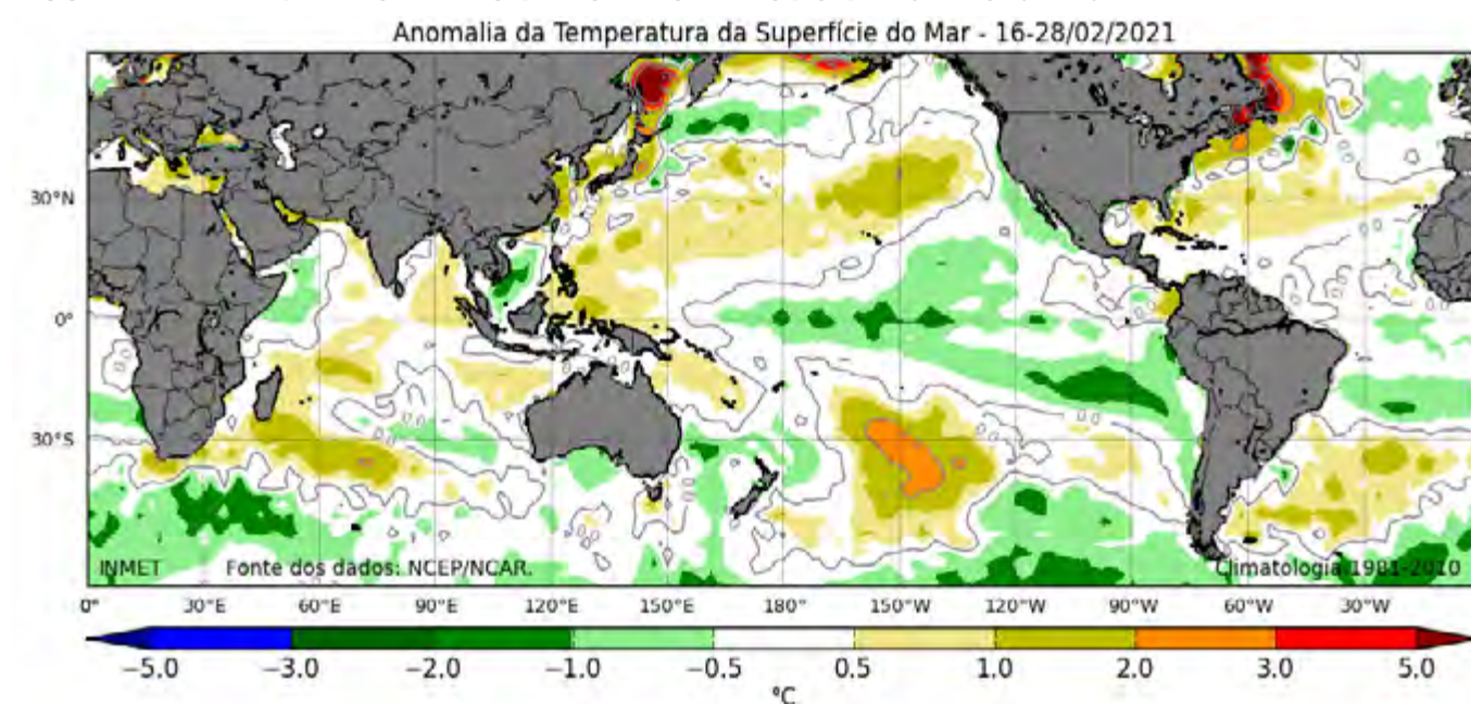
FIGURA 2 - MAPA DE ANOMALIAS DA TSM NO PERÍODO DE 16 A 28/02/2021
