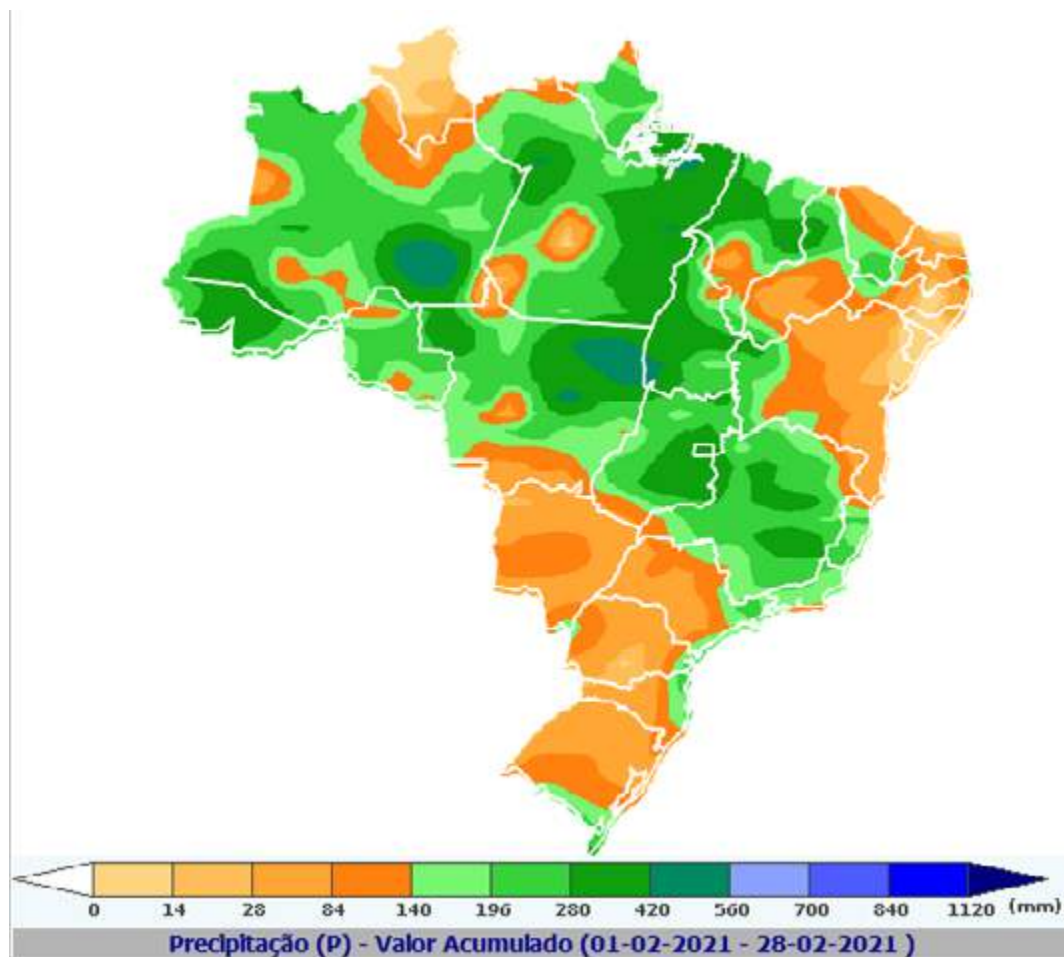
FIGURA 1 - MAPAS DE PRECIPITAÇÃO ACUMULADA EM FEVEREIRO/2021
