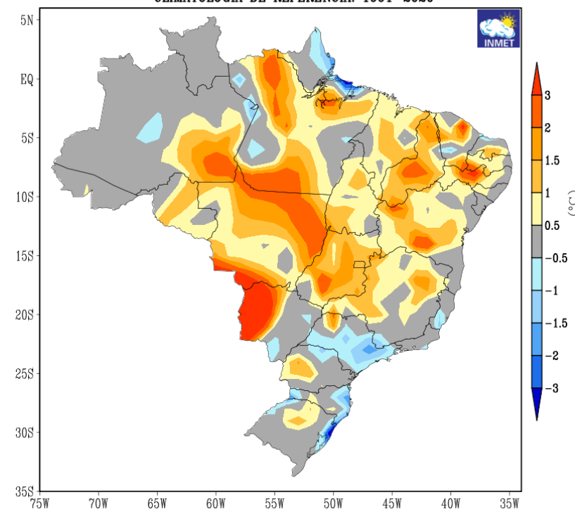
ANOMALIAS DE TEMPERATURAS MÉDIAS VALIDO NOVEMBRO de 2025 CLIMATOLOGIA DE REFERENCIA: 1991-2020
