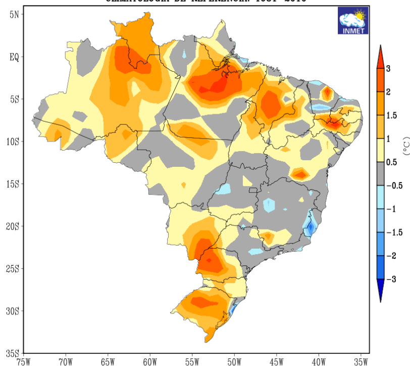
ANOMALIAS DE TEMPERATURAS MÉDIAS VALIDO NOVEMBRO de 2024 CLIMATOLOGIA DE REFERENCIA: 1981-2010
