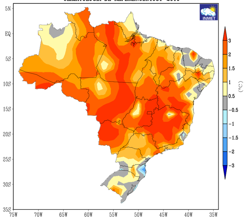
ANOMALIAS DE TEMPERATURAS MÉDIAS VALIDO PARA NOVEMBRO DE 2023 CLIMATOLOGIA DE REFERENCIA: 1981-2010
