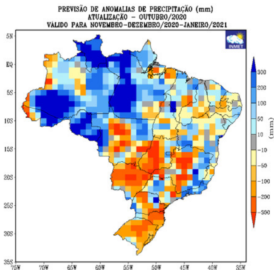
FIGURA 3 - PREVISÃO PROBABILÍSTICA DE PRECIPITAÇÃO PARA O TRIMESTRE NOVEMBRO-DEZEMBRO/2020 E JANEIRO/2021
