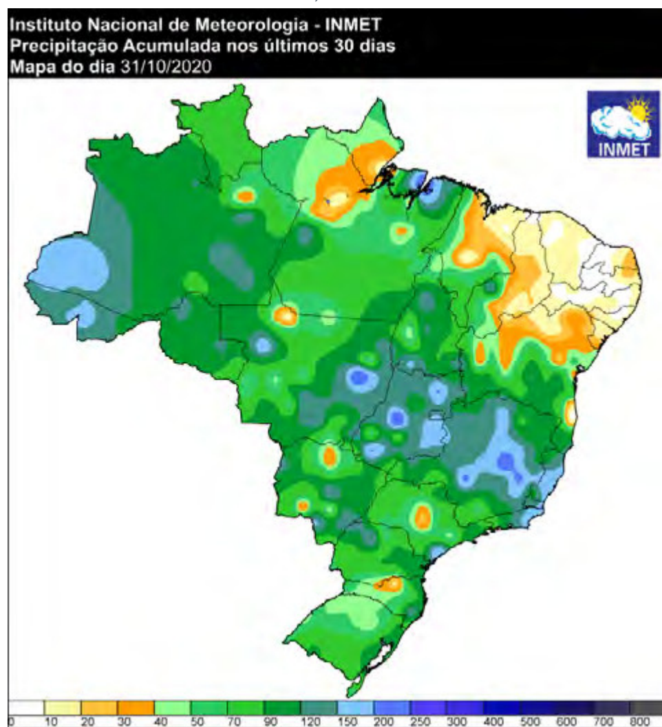
FIGURA 1 - MAPAS DE PRECIPITAÇÃO ACUMULADA EM OUTUBRO/2020
