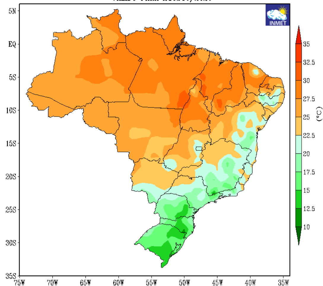
TEMPERATURA MÉDIA PREVISTA (°C) ATUALIZACAO - JULHO/2026 VALIDO PARA AGOSTO/2026
