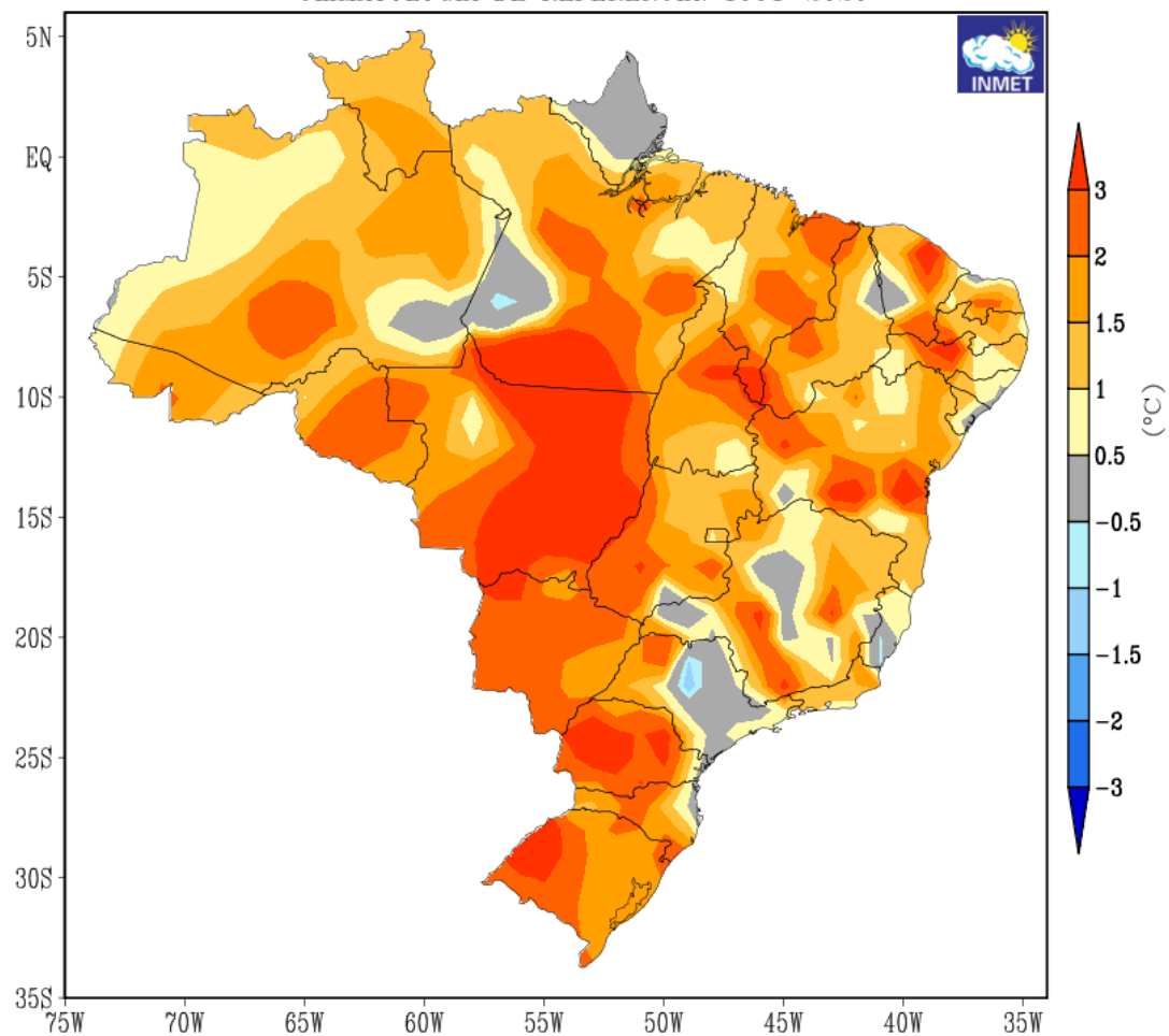
ANOMALIAS DE TEMPERATURAS MÉDIAS VALIDO JULHO de 2026 CLIMATOLOGIA DE REFERENCIA: 1991-2020
