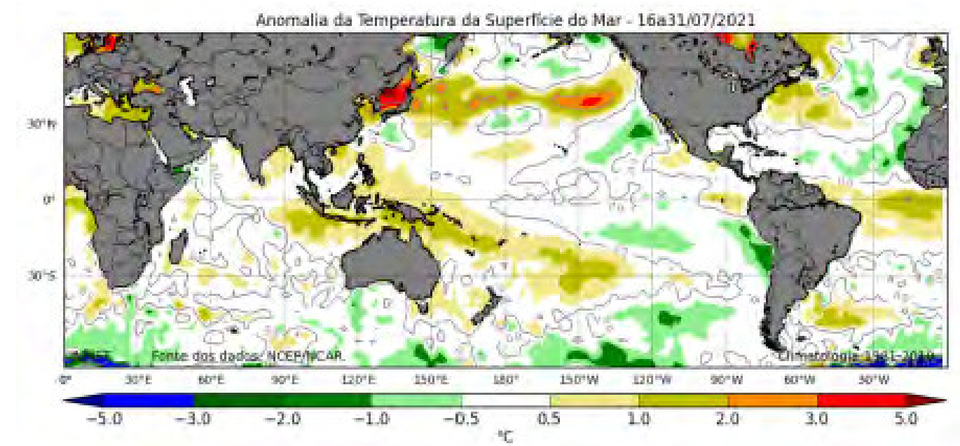
FIGURA 3 - MAPA DE ANOMALIAS DA TSM NO PERÍODO DE 16 A 31/7/2021
