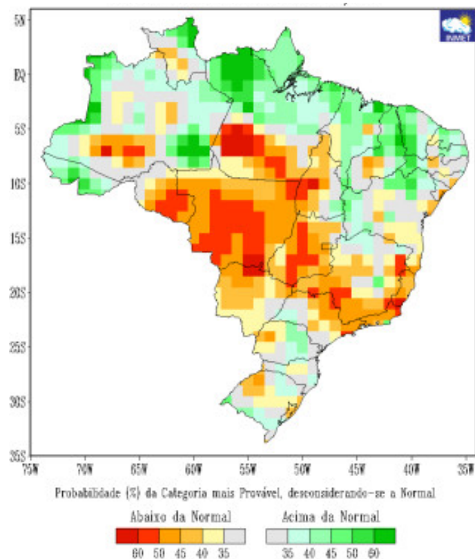
FIGURA 5 - PREVISÃO PROBABILÍSTICA DE PRECIPITAÇÃO PARA O TRIMESTRE AGOSTO-SETEMBRO-OUTUBRO/2021
