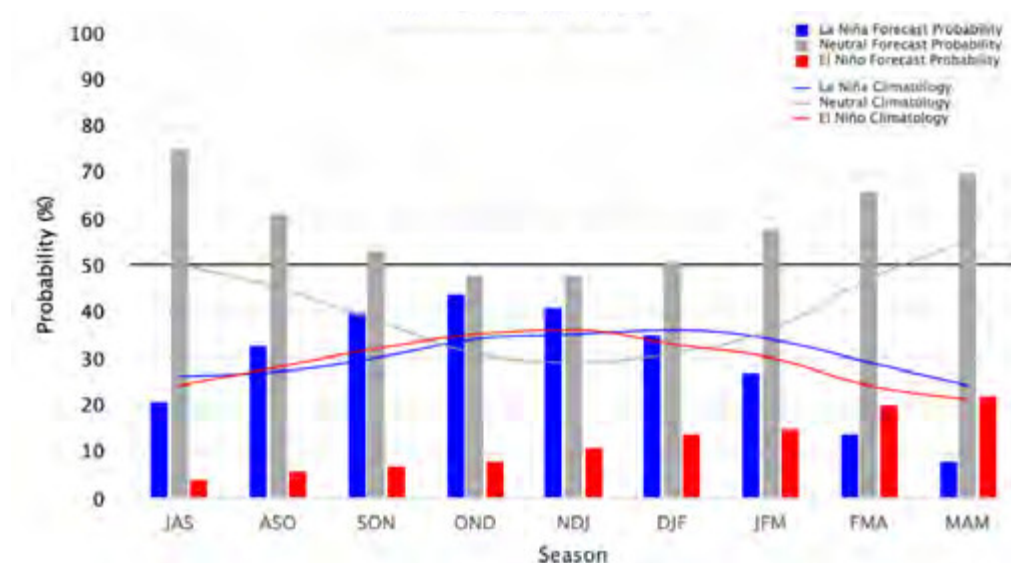
GRÁFICO 1 - PREVISÃO PROBABILÍSTICA DO IRI PARA OCORRÊNCIA DE EL NIÑO OU LA NIÑA
