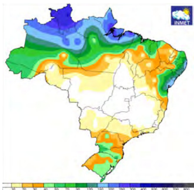
FIGURA 1 - MAPA DE PRECIPITAÇÃO ACUMULADA EM JULHO DE 2021
