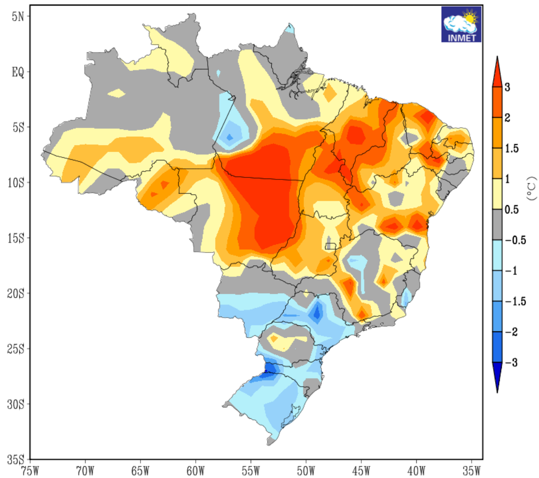
ANOMALIAS DE TEMPERATURAS MÉDIAS VALIDO JUNHO de 2026 CLIMATOLOGIA DE REFERÊNCIA: 1991-2020
