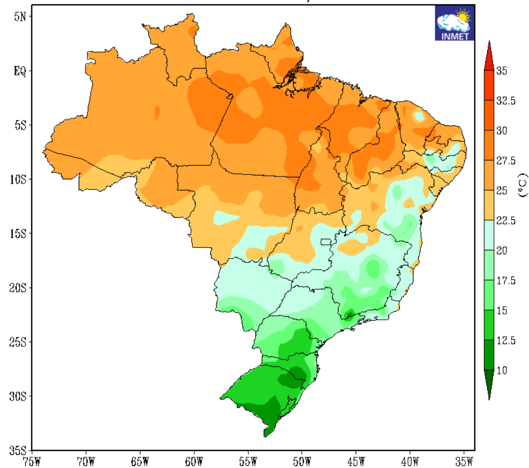
TEMPERATURA MÉDIA PREVISTA (°C) ATUALIZAÇÃO - JUNHO/2026 VALIDO PARA JULHO/2026
