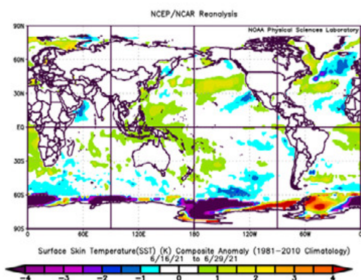
FIGURA 2 - MAPA DE ANOMALIAS DA TSM NO PERÍODO DE 16 A 29/6/2021
