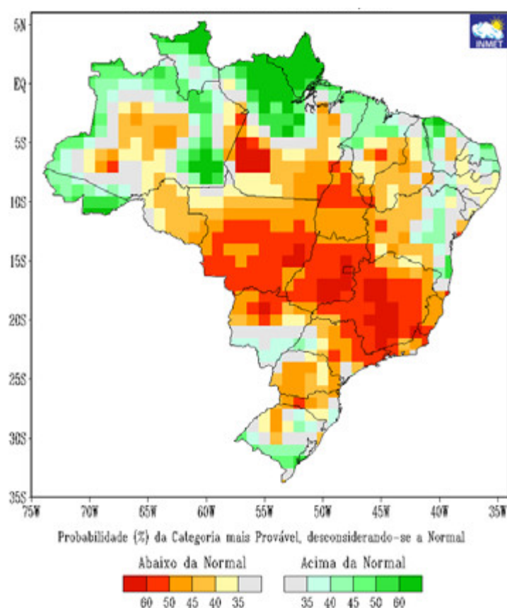
FIGURA 5 - PREVISÃO PROBABILÍSTICA DE PRECIPITAÇÃO PARA O TRIMESTRE JULHO-AGOSTO-SETEMBRO/2021
