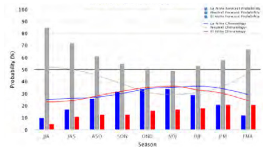
FIGURA 4 - PREVISÃO PROBABILÍSTICA DO IRI PARA OCORRÊNCIA DE EL NIÑO OU LA NIÑA
