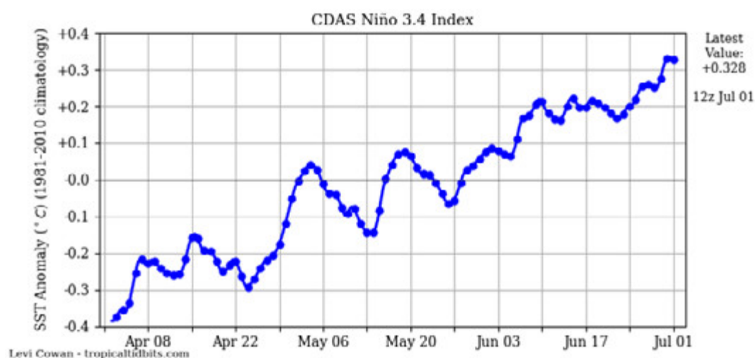
FIGURA 3 - GRÁFICO DE MONITORAMENTO DO ÍNDICE DIÁRIO DE EL NIÑO/LA NIÑA NA REGIÃO 3.4
