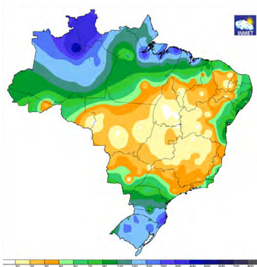
FIGURA 1 - MAPA DE PRECIPITAÇÃO ACUMULADA EM JUNHO DE 2021
