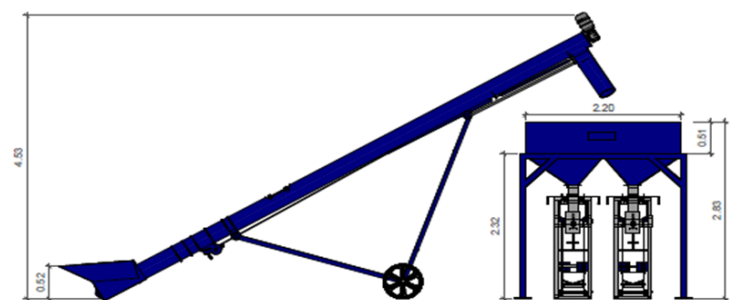
VISTA LATERAL 1 1:20
