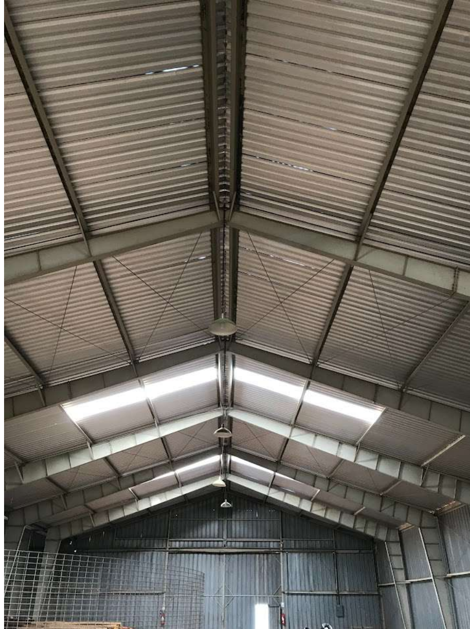
Tesouras onde serão ancorados com vãos de 6 m.
