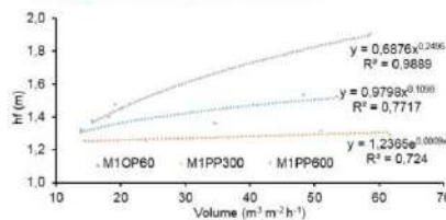
Figura 3. Perda de carga (hf) para diferentes taxas de filtragem utilizando água limpa com uma camada de MSNT antes e uma depois da camada de carvão ativado de 0,15 m (CaAt).
