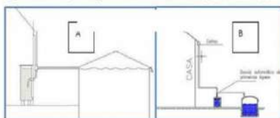
Figura 1 - Desvio das primeiras águas de chuva: Vasos Comunicantes (A); Fecho Hídrico (B).
