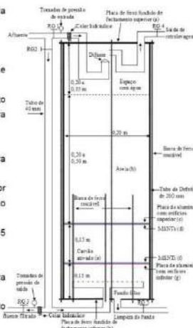
Figura 1. Módulo experimental.
