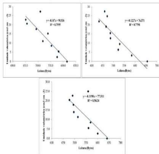
Figura 1. Figura 1 Curva de calibração obtida em laboratório do sensor YL69 para o Gleissolo.
