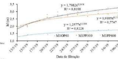
Figura 5. Perda de carga (hf) com taxa de filtração 60 m³ m⁻² h⁻¹ de EET por SZR e uma camada MSNT antes e uma depois da camada de carvão ativado de 0,30 m e areia de 0,60 m.
