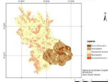
Figura 3- Mapa de suscetibilidade à erosão do Município de Grupiara-MG
