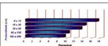
Figura 1. Percentagem de Saturação de Bases em Profundidade no Perfil de Solo
