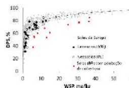
Fig.3: Efeito de grãos de adubo no valor de WSP (BR = Brasil)
