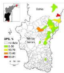
Fig.2: Grau de saturação de fósforo em solos do alto São Francisco
