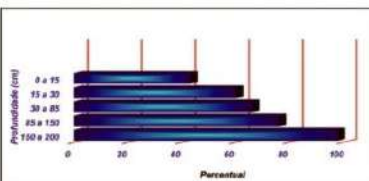
Figura 2. Saturação de Alumínio em Profundidade no Perfil de Solo
