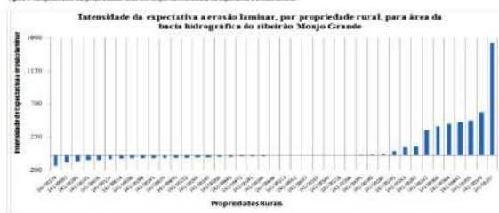
Figura 4. Mapeamento das propriedades rurais em função da intensidade da expectativa e modelização.
