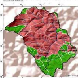
Figura 3. Detecção de propriedades rurais com perdas de solo acima dos limites naturalmente toleráveis.
