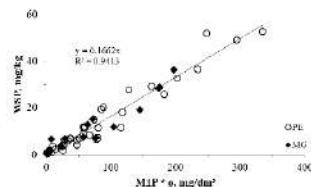
Fig.1: Correlação entre M1P e WSP em amostras de solo de Minas Gerais (MG) e Pernambuco (PE); locais de amostragem nos solos são indicados com círculos (Fig.2); (unidades de medida: M1P: mg/kg; q: kg/cm 3 )
