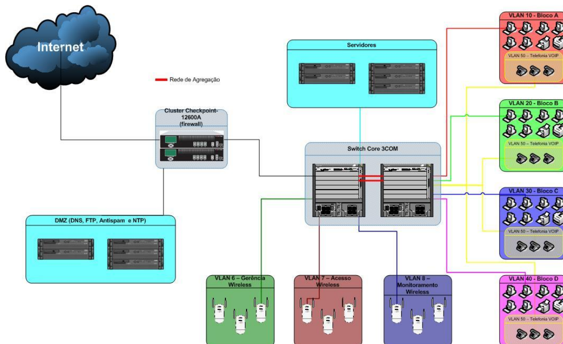
Figura 14 – Rede e serviços
