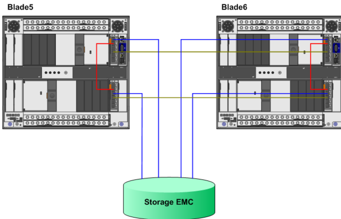
Figura 21 – Rede SAN de IBM Blade 5 e 6
