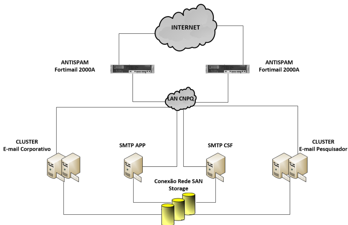
Figura 15 – Rede de Serviços de E-mail
