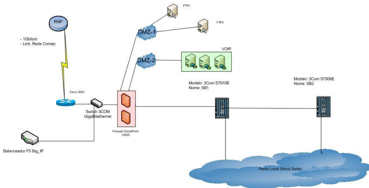
Figura 12 – Diagrama Geral da Rede CNPq
