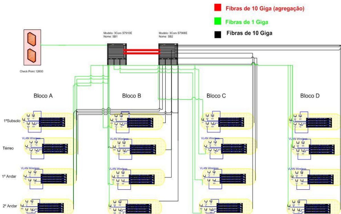
Figura 13 – Diagrama de Interconexão de Rede
